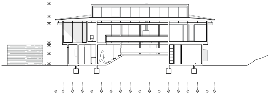
CORTE 1 - 1
