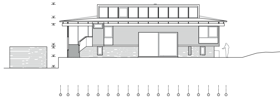
ELEVACIÓN ORIENTE
