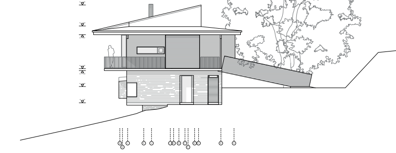
ELEVACIÓN SUR
