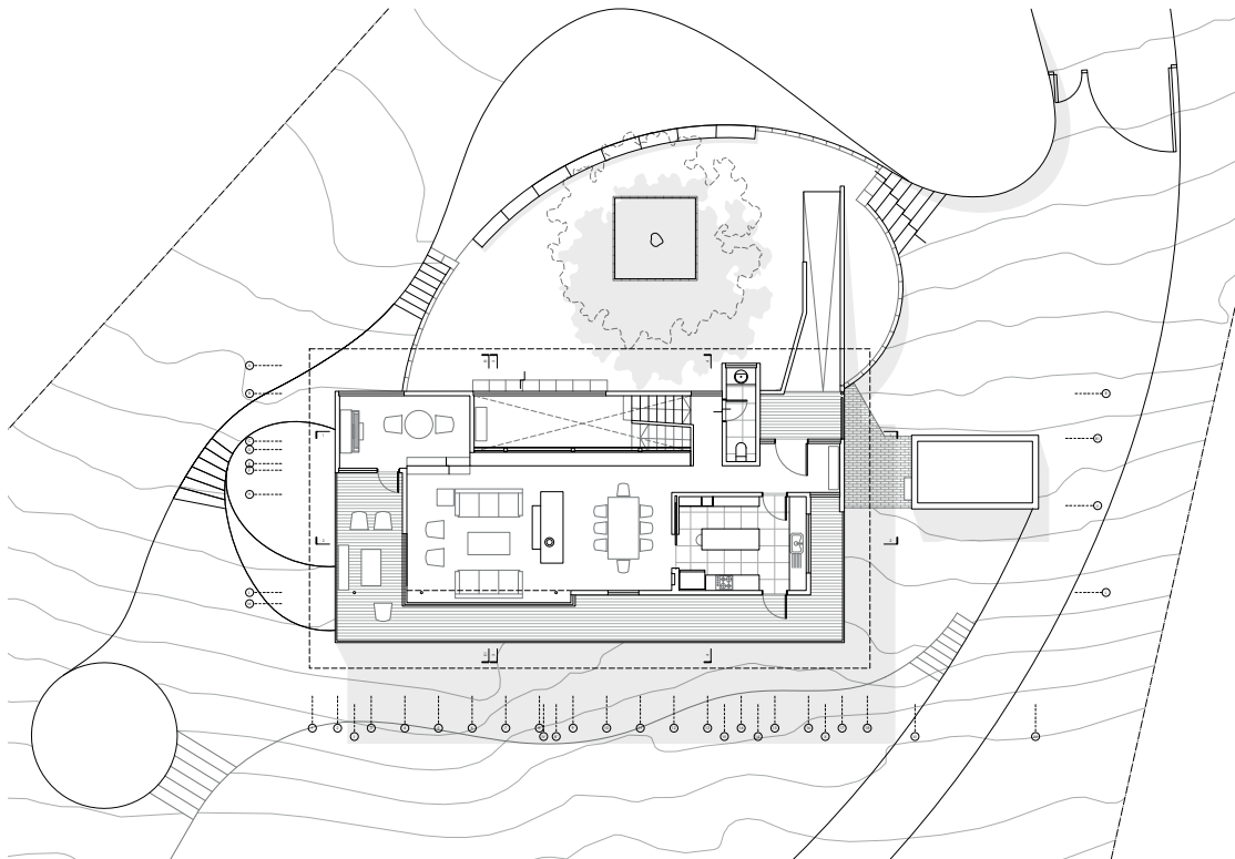
PLANTA PISO 2
