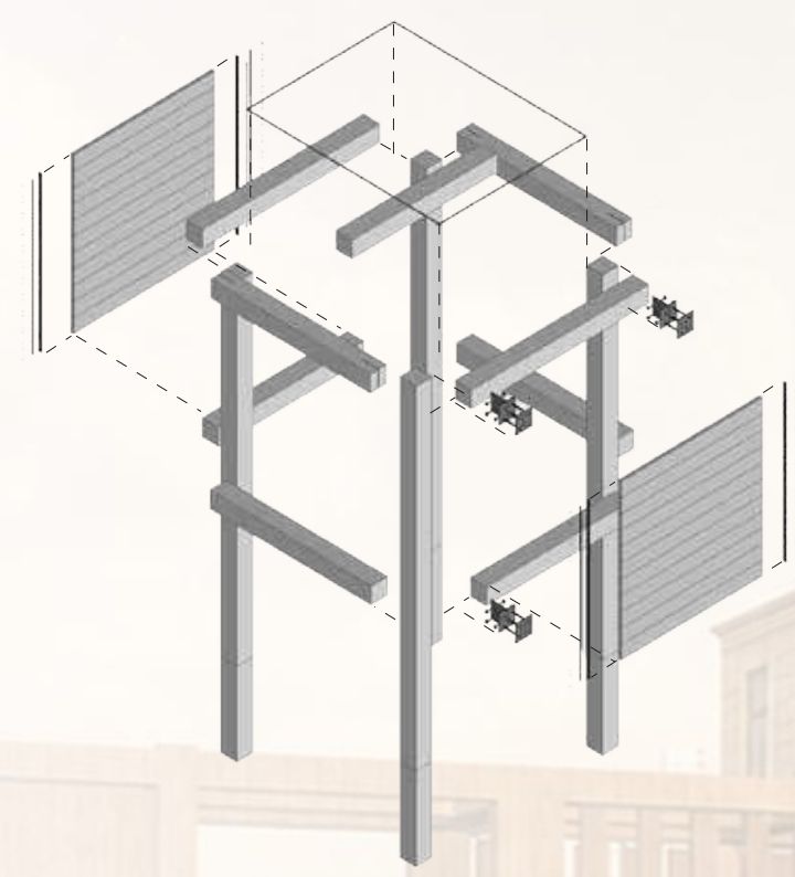
EXPLOTADA DETALLE
