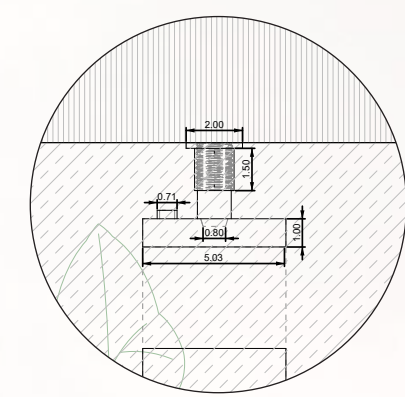
DETALLE UNIÓN ESC: S/E
