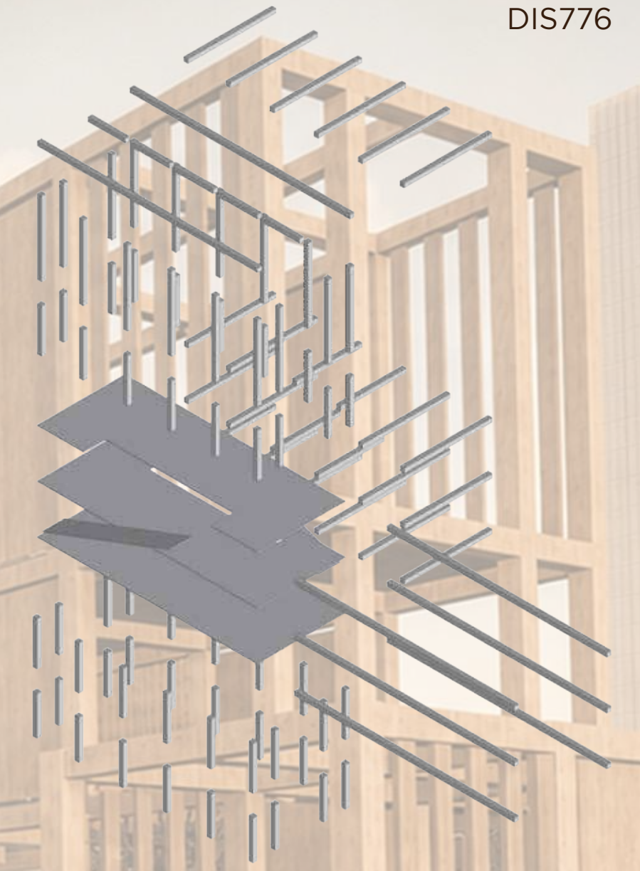
EXPLOTADA TORRE
