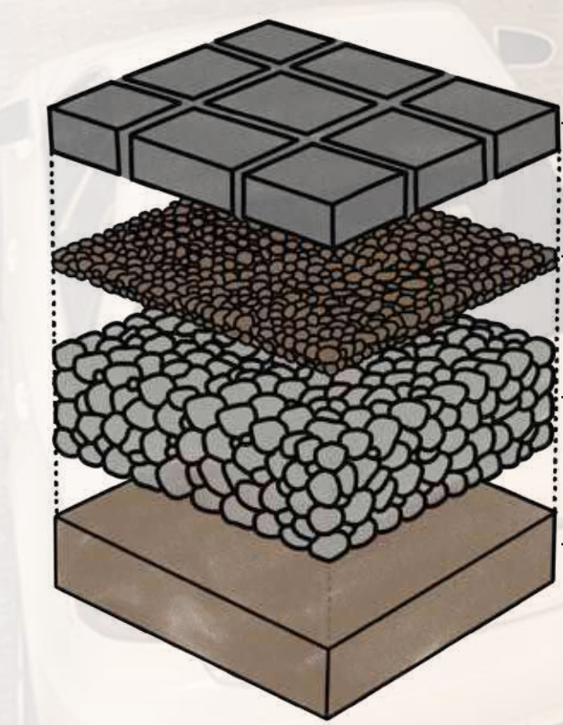
BASE HORMIGÓN
