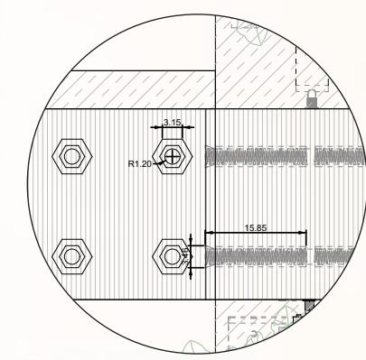
DETALLE RIEL 1 ESC: S/E
