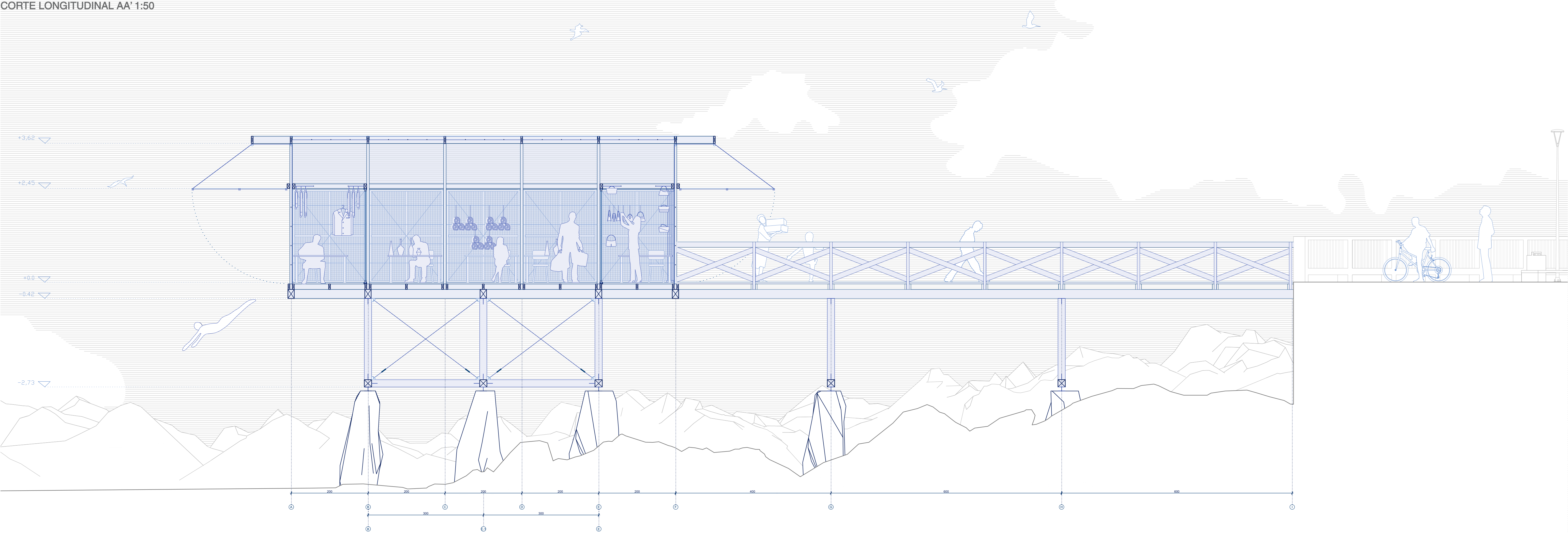
CORTE LONGITUDINAL AA' 1:50
