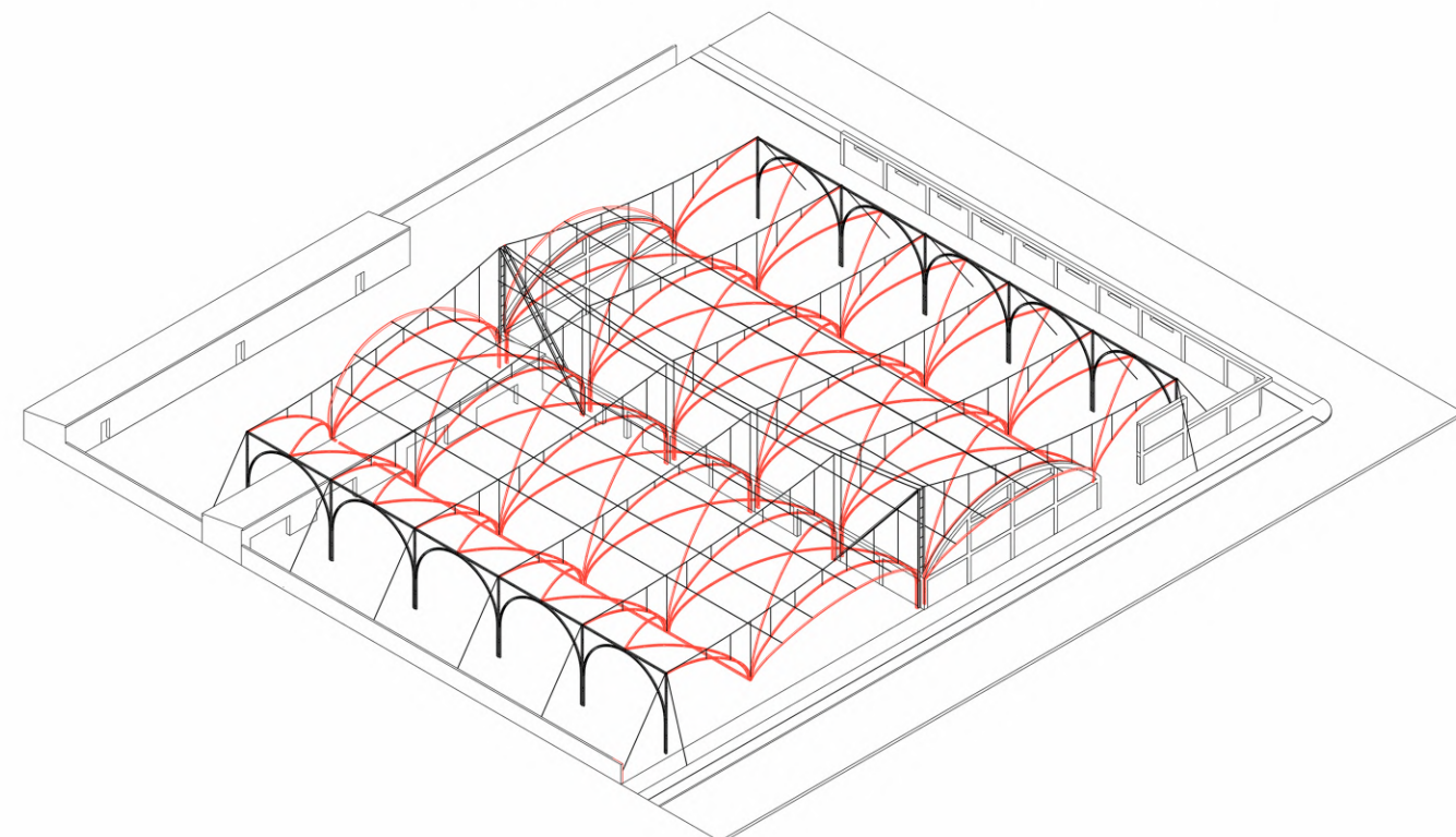
5- LEVANTAMIENTO ARCOS INTERIORES
