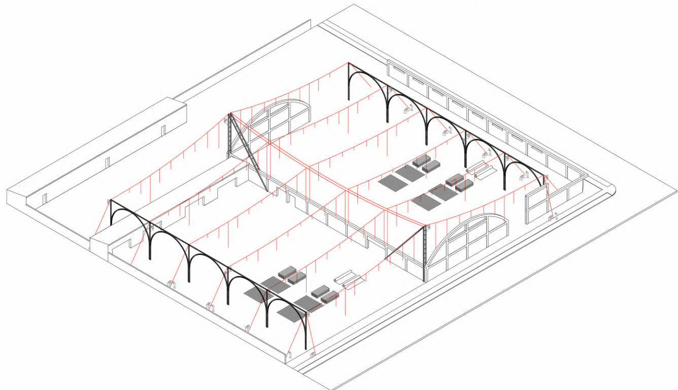
6- LEVANTAMIENTO CUBIERTA POLIETILENO RECICLADO
