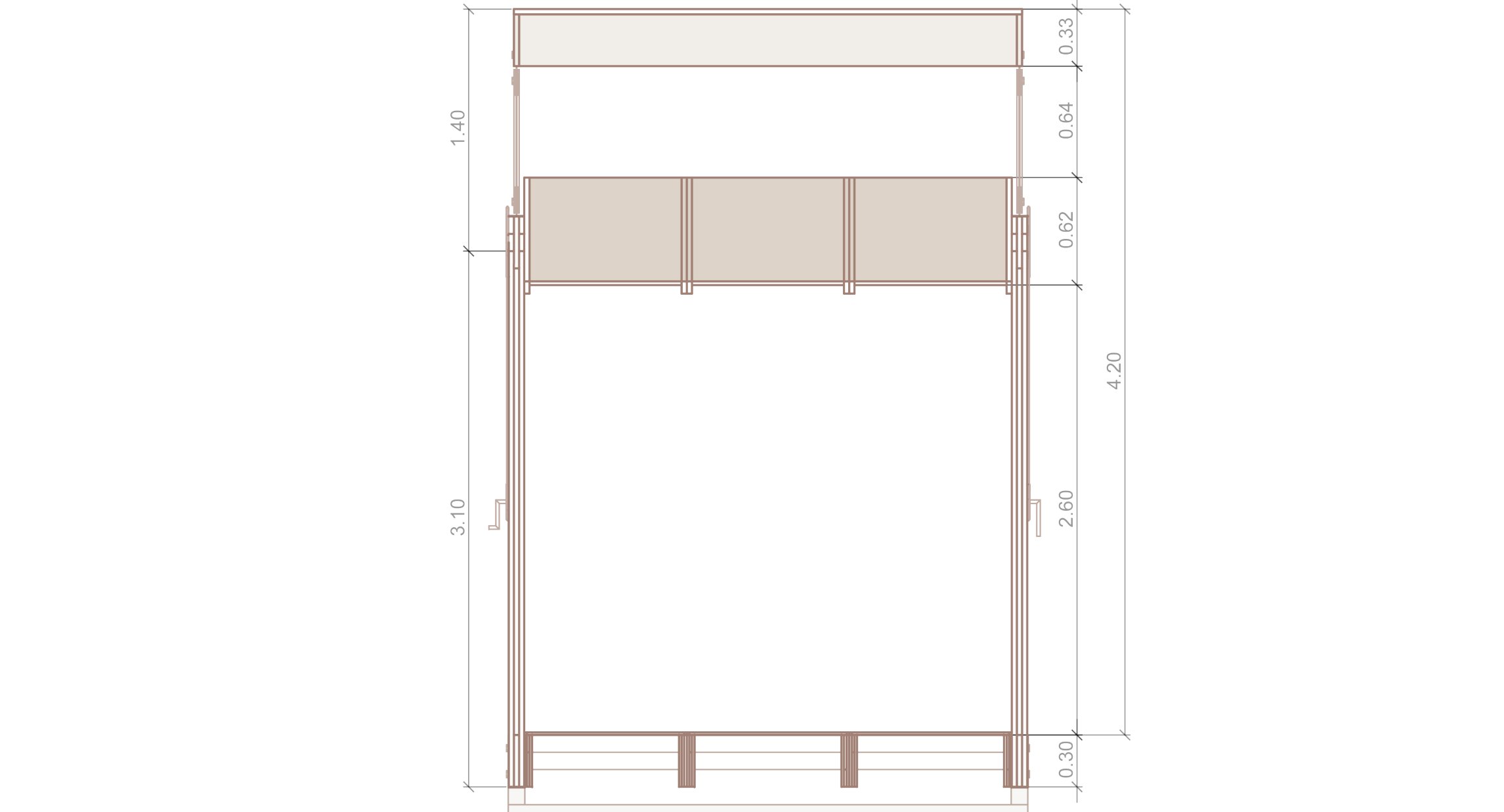
VISTA LATERAL
