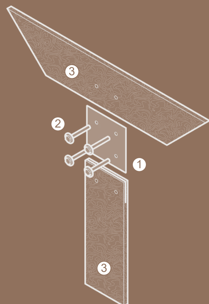
A UNIÓN MONTANTE - VIGA
