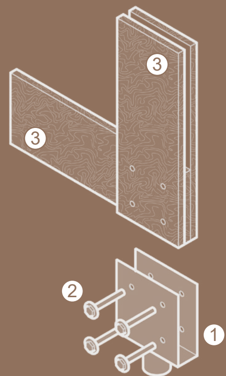
B UNIÓN COLUMNA - BASE
