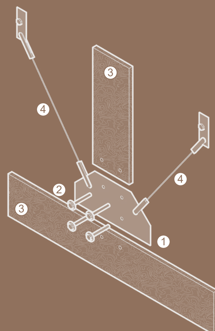
D PLATINA Y TENSORES
