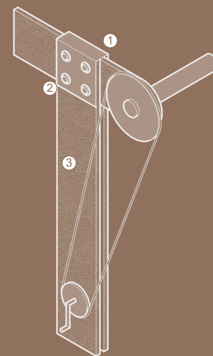
E DETALLE DE POLEA
