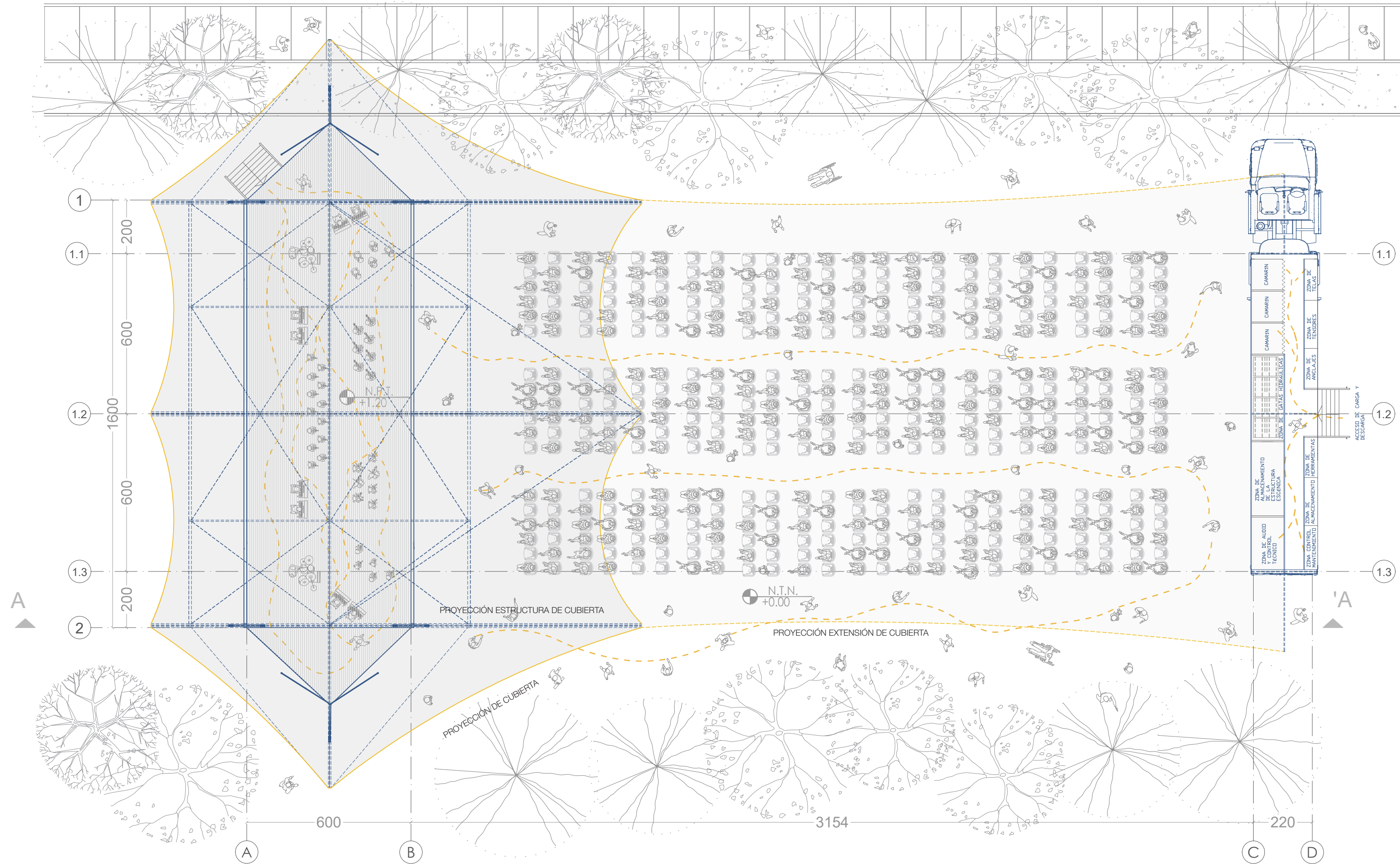
PLANTA GENERAL - ORQUESTA INFANTIL ESC. 1:125
