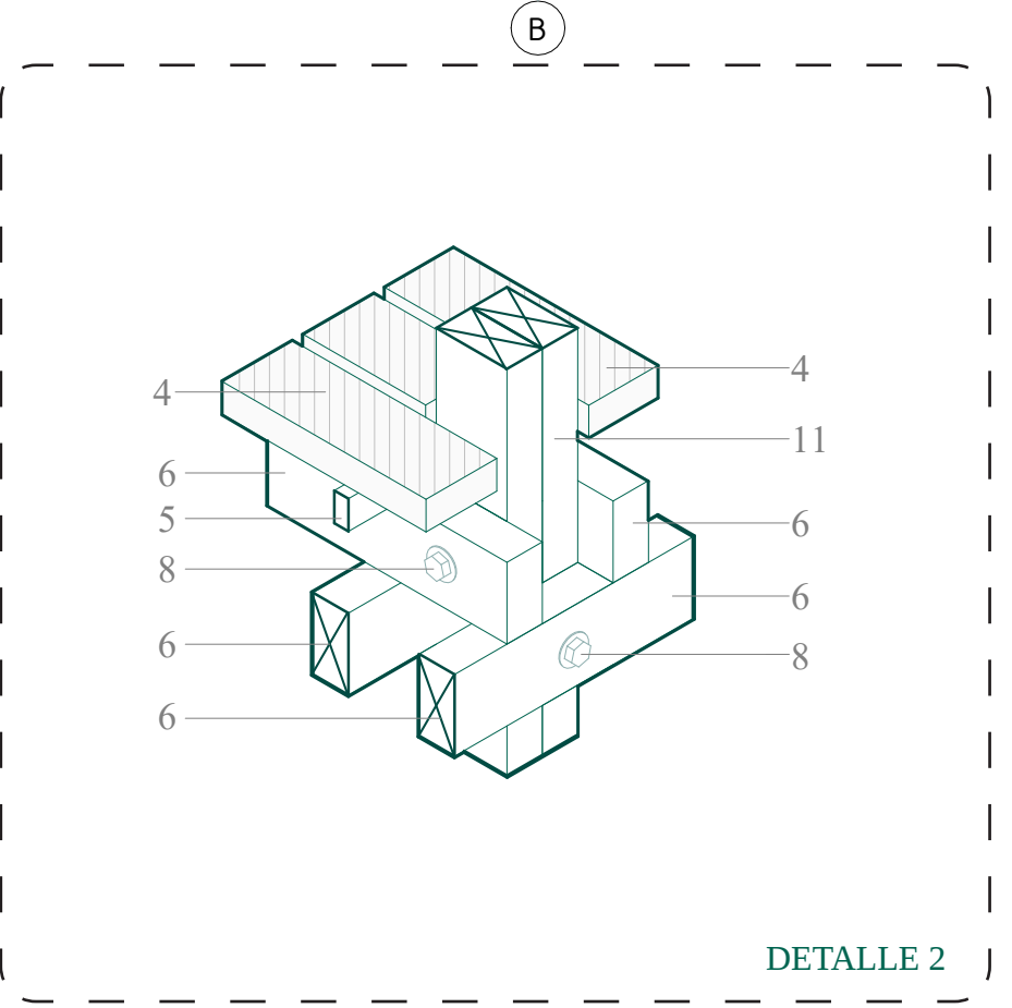
Escantillón Fugado esc 1:25
