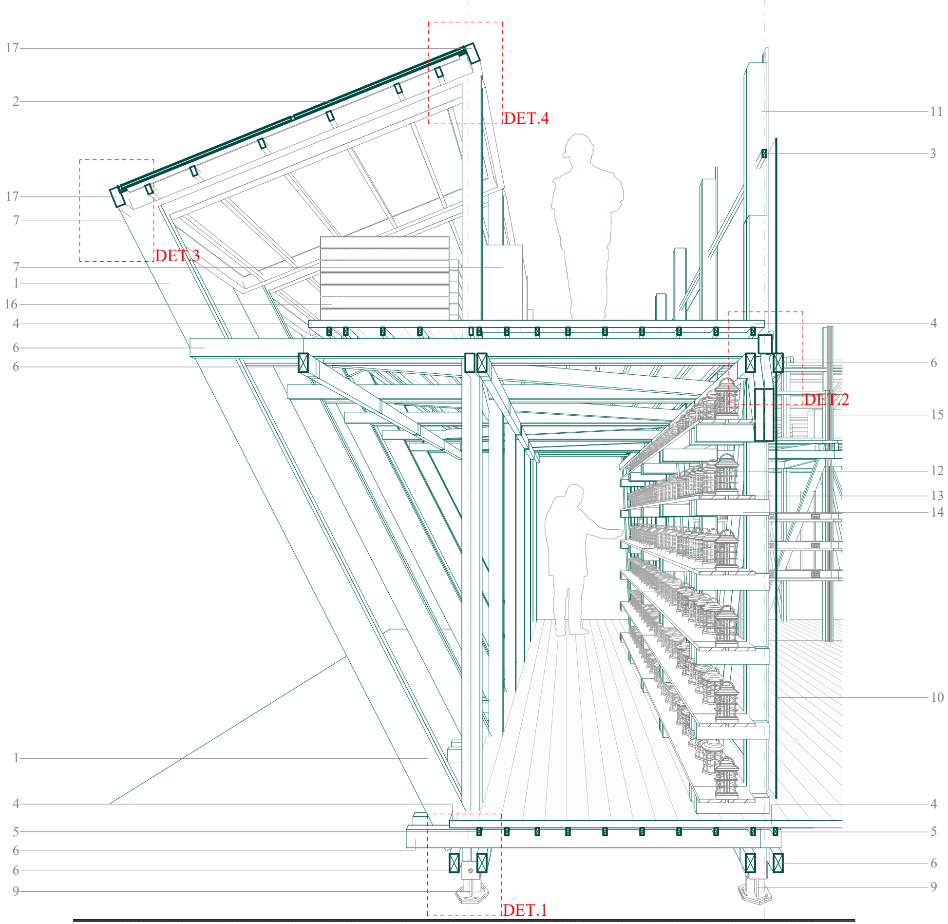
Escantillón Fugado esc 1:25
