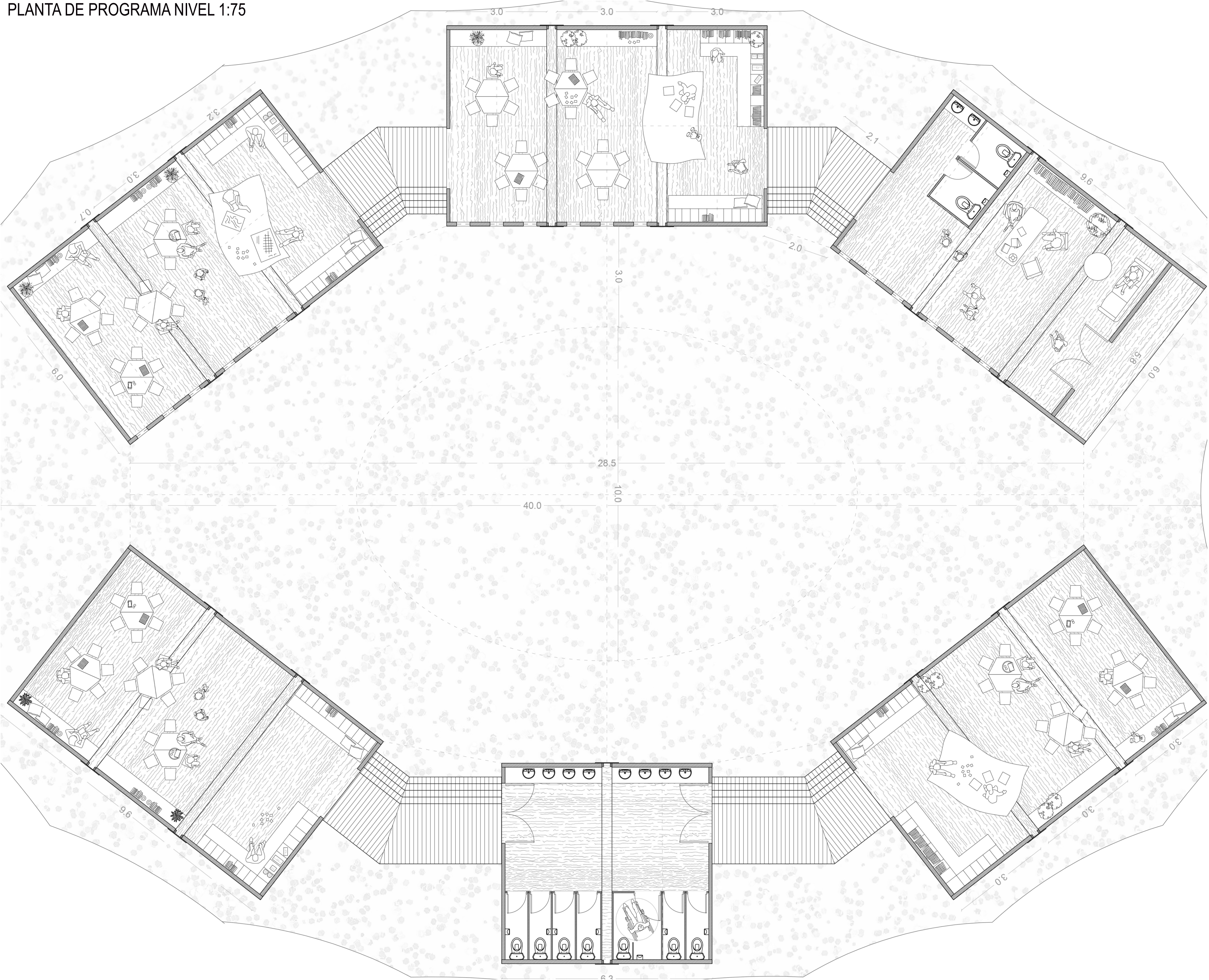
PLANTA DE PROGRAMA NIVEL 1:75
