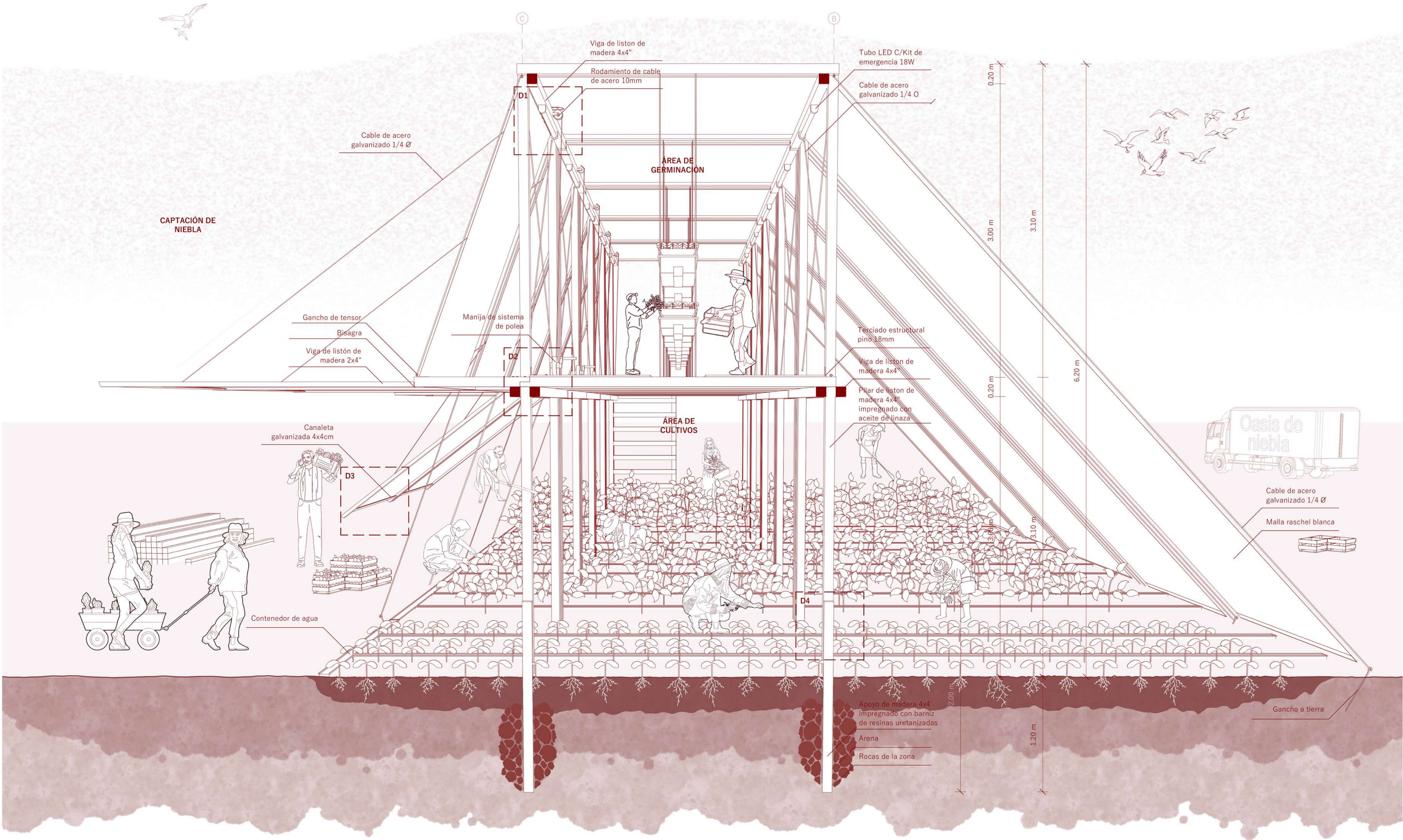
CORTE PERSPECTIVADO ESC 1:25
