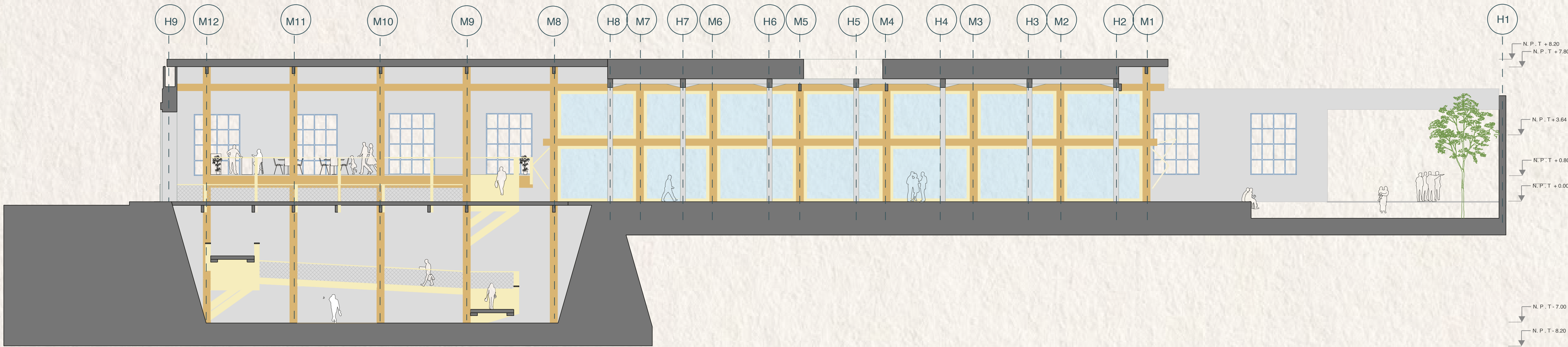
Corte longitudinal Escala 1:100
