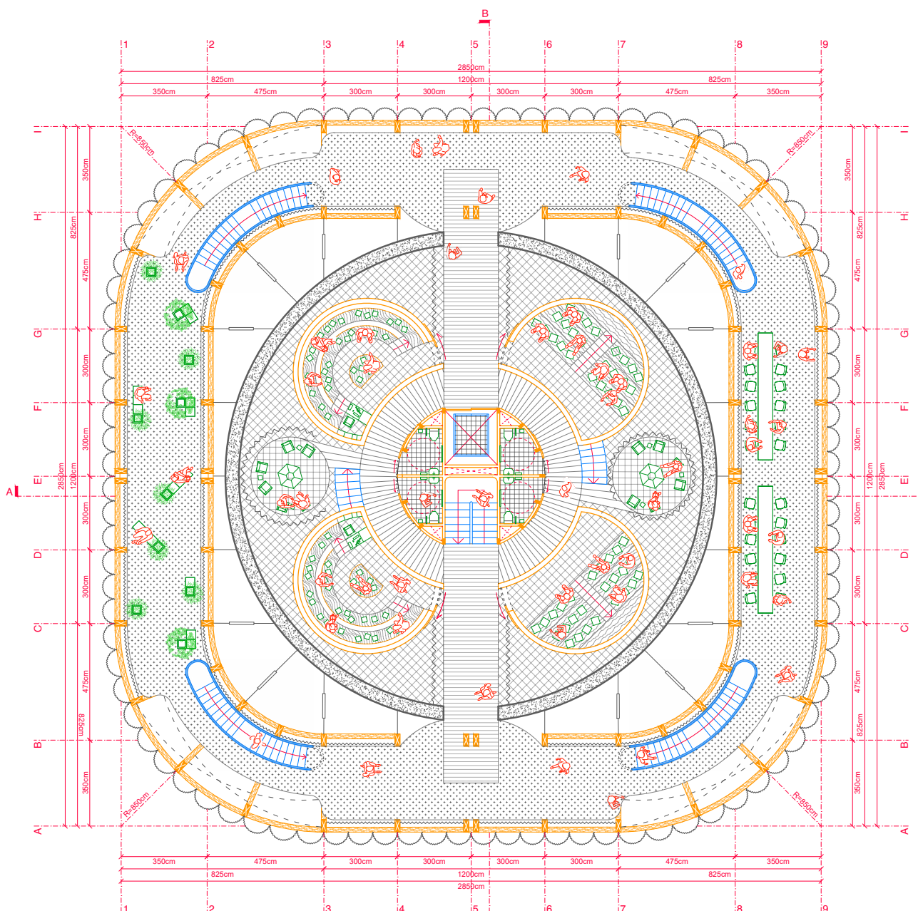
PLANTA ESTANQUE ESCALA 1:200
