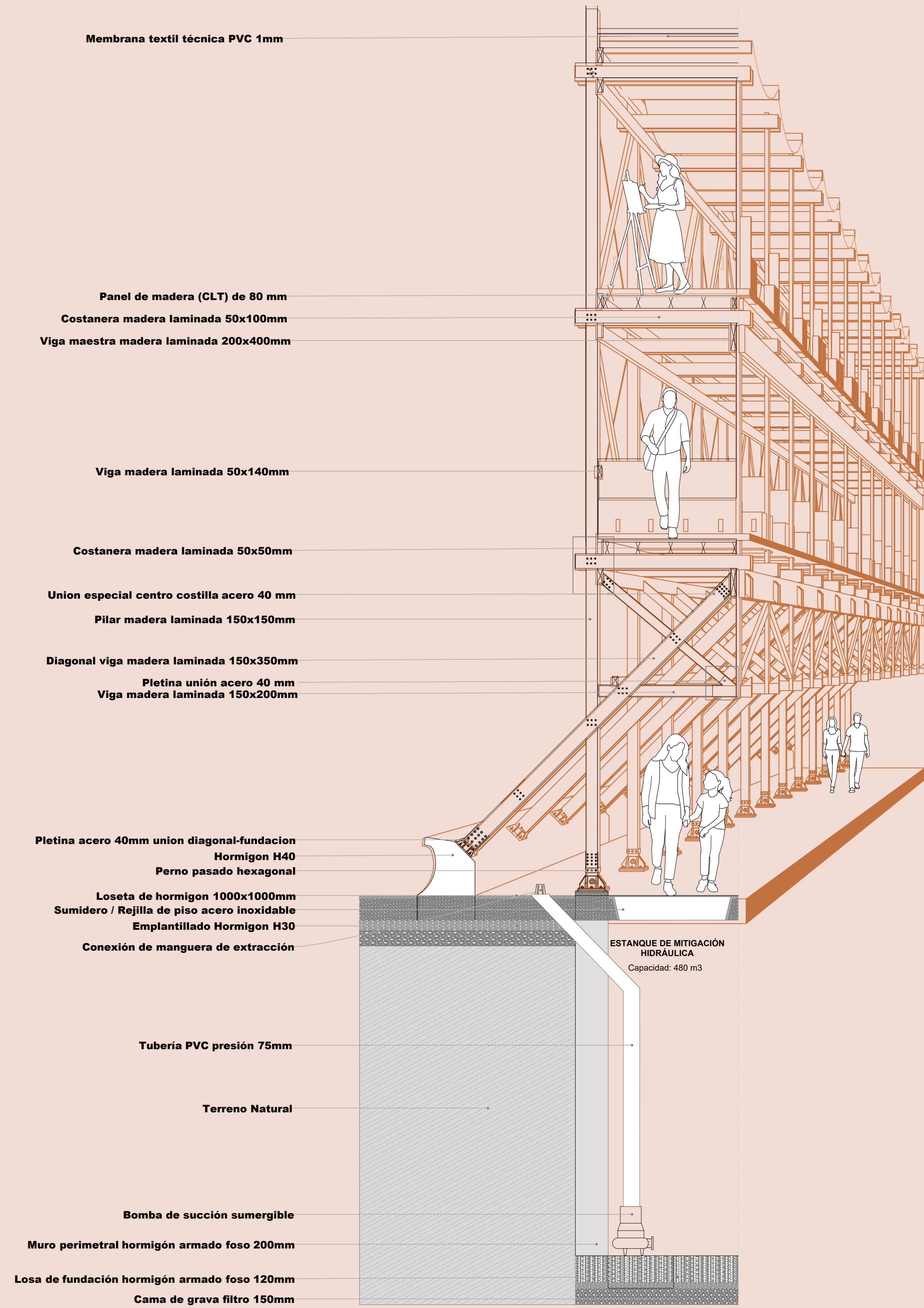
Escantillón ESQ 1:35
