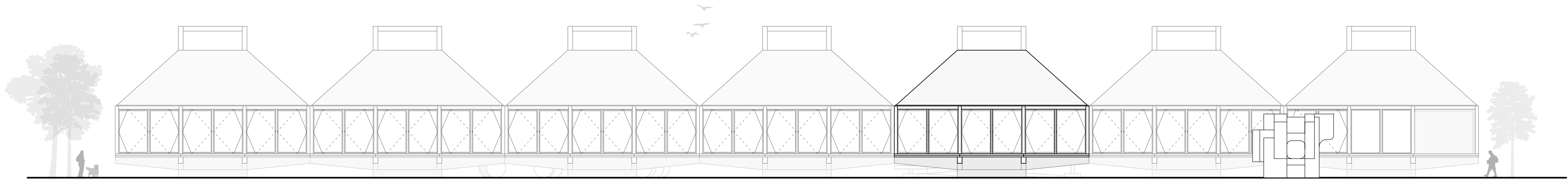
Elevación suroeste Esc. 1:200
