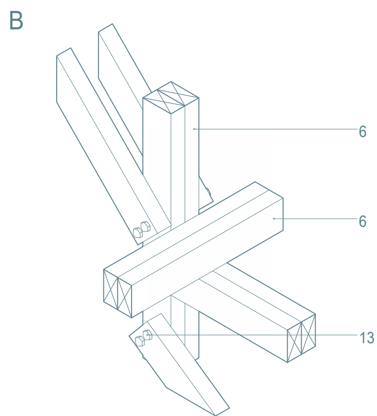
Detalle Escantillón B. Escala 1:5
