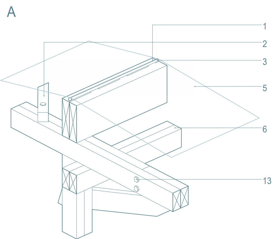
Detalle Escantillón A. Escala 1:5
