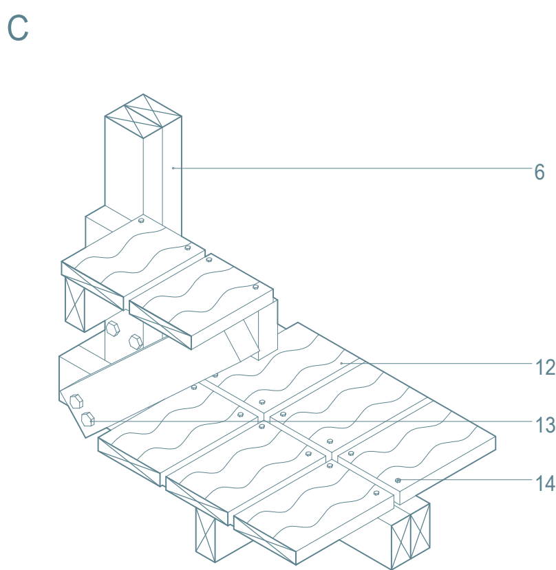
Detalle Escantillón C. Escala 1:5
