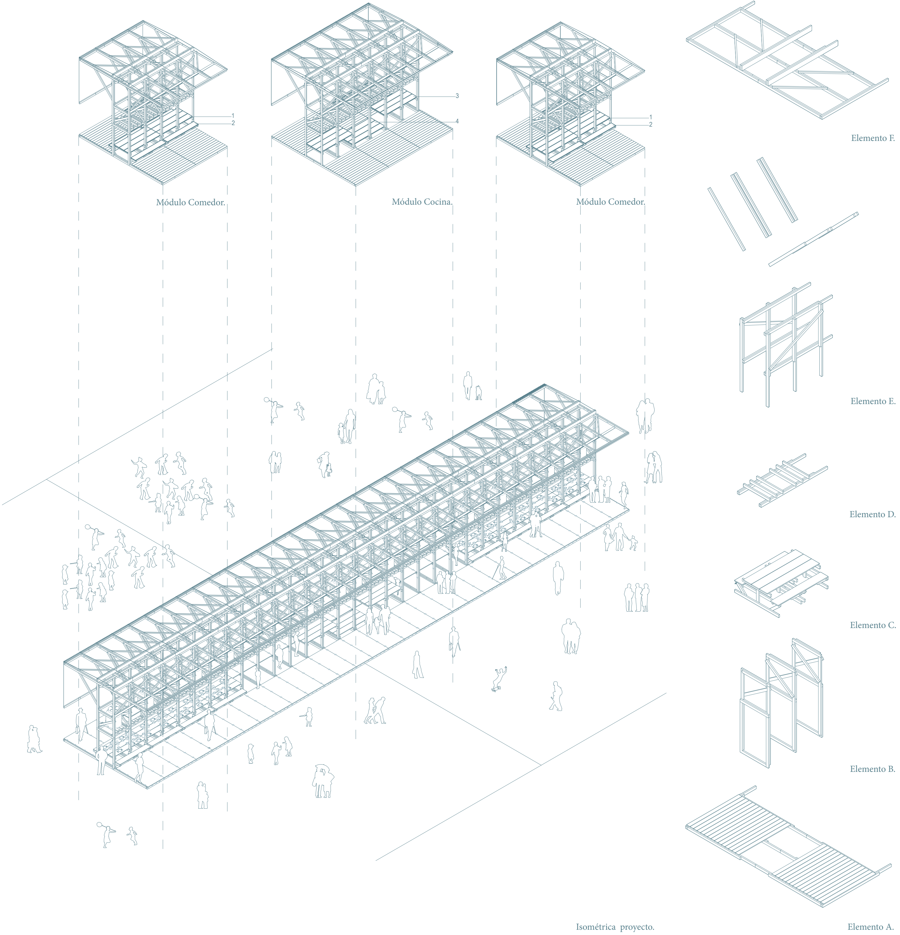
Isométrica proyecto.
