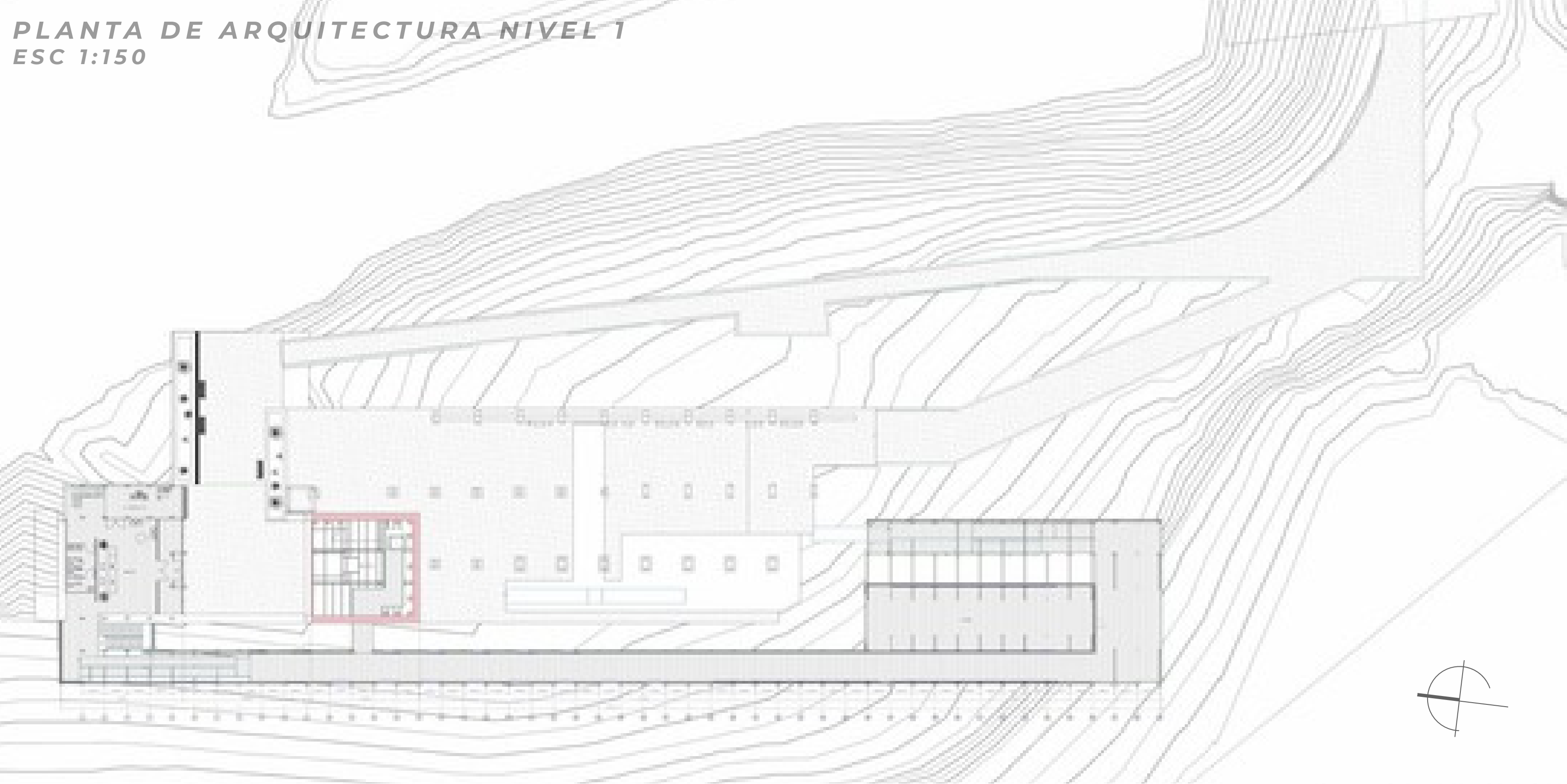
PLANTA DE ARQUITECTURA NIVEL -1 ESC 1:150
