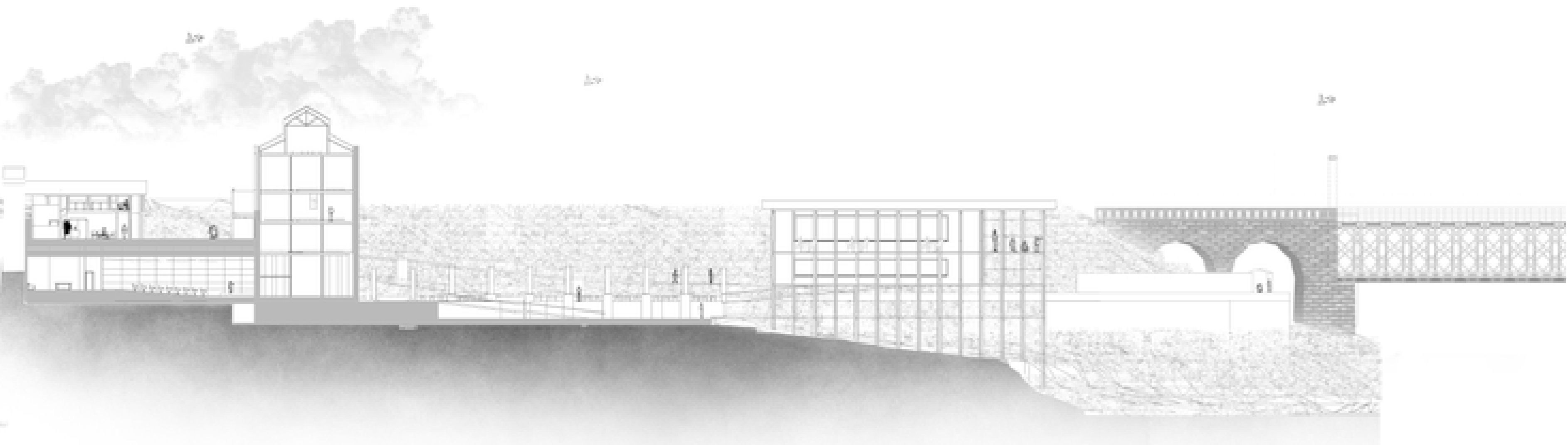
CORTE LONDIGTUCINAL ESC 1:150
