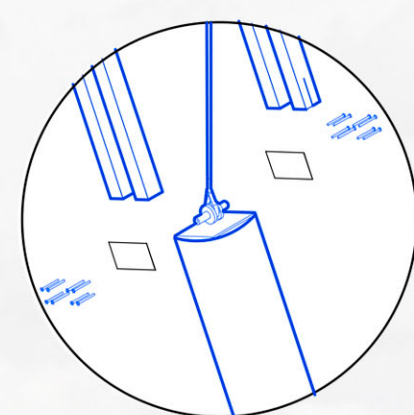
Detalles | Esc. 1: 50
