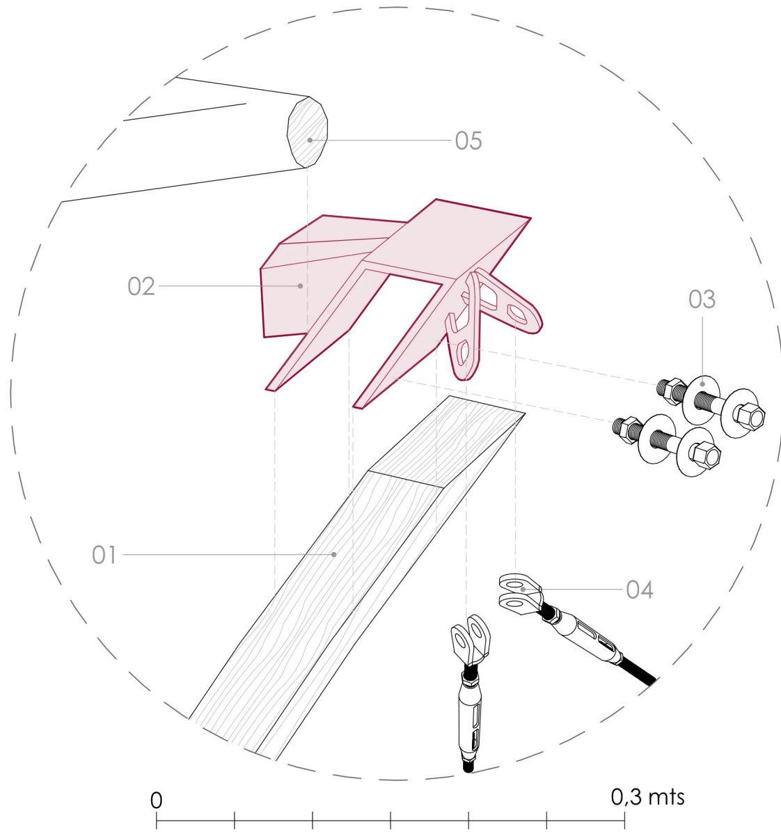
DETALLE 04 | UNIONES TENSOR Y CILINDRO
