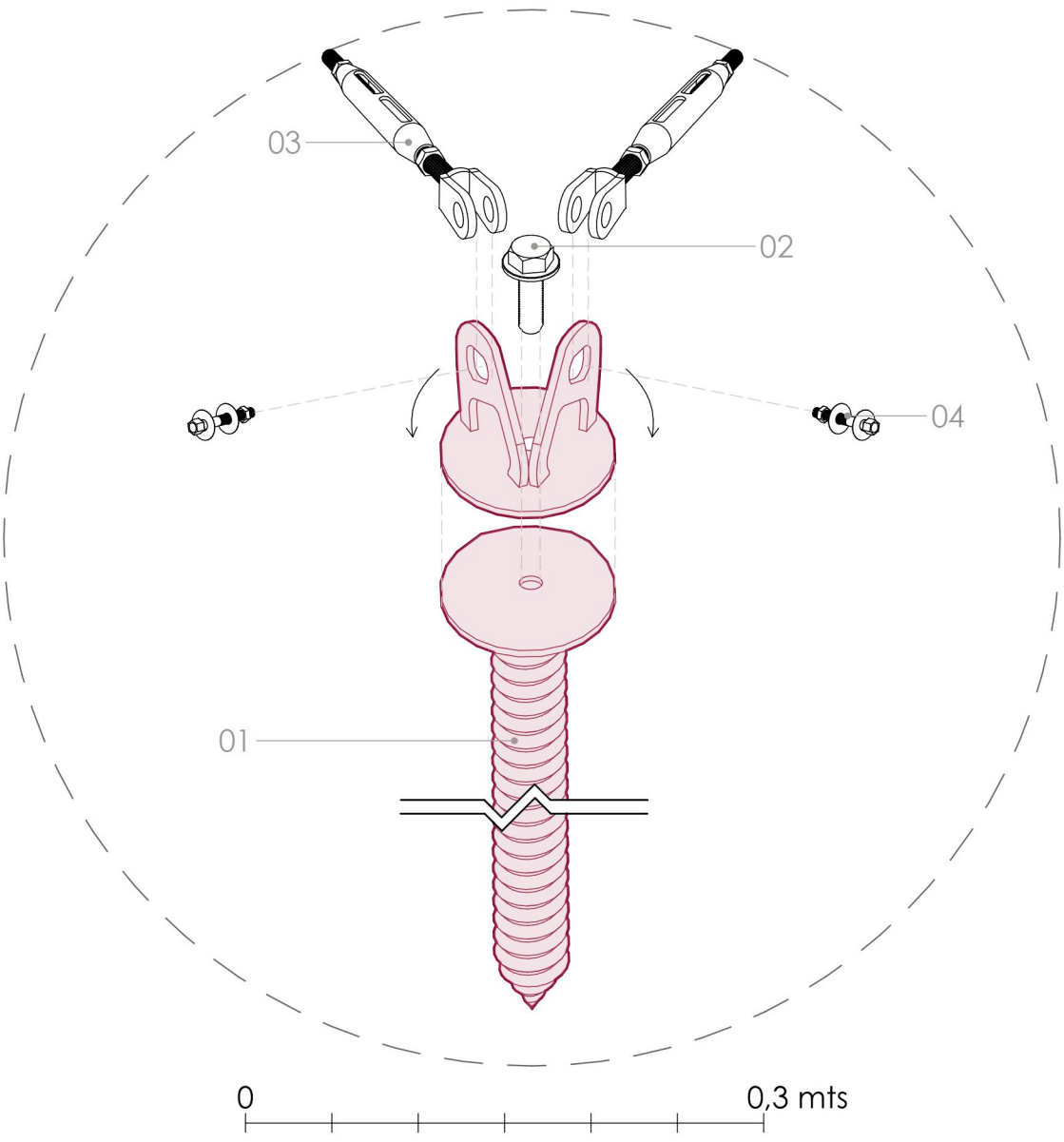
DETALLE 01 | ANCLAJE TENSOR A SUELO
