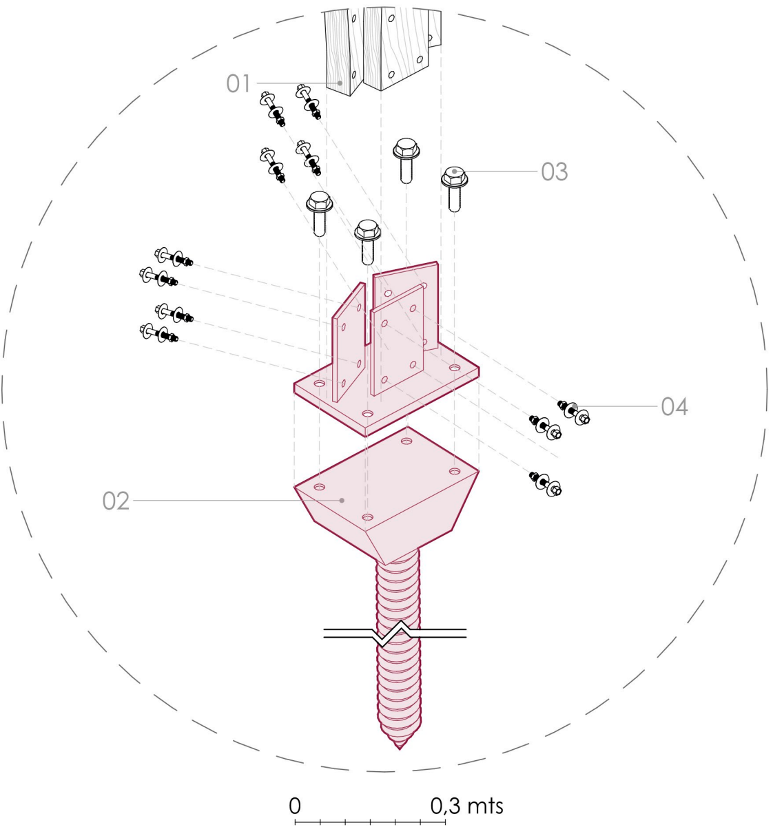
DETALLE 02 | ANCLAJE PILAR A SUELO
