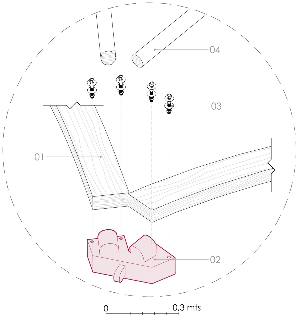
DETALLE 05 | UNIONES SEPARADOR Y HERRAJE
