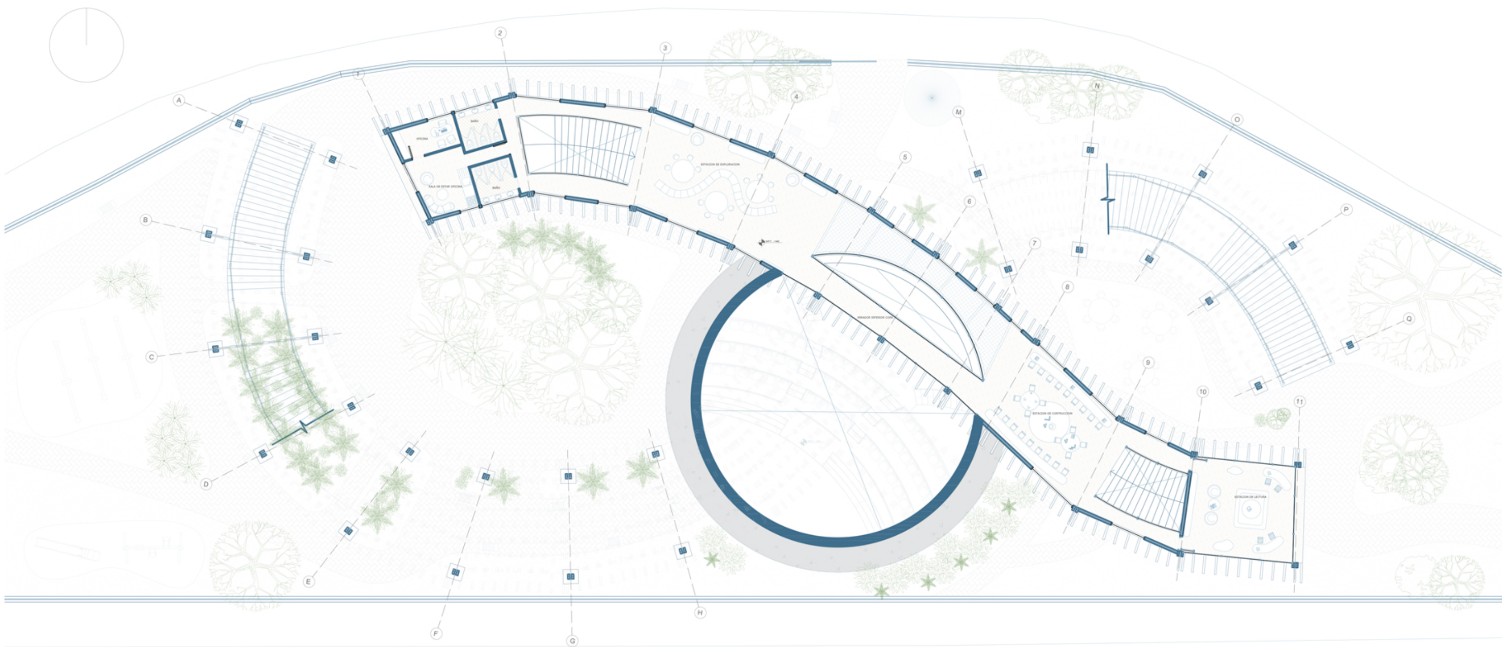
PLANTA NIVEL 2 Esc. 1 : 200
