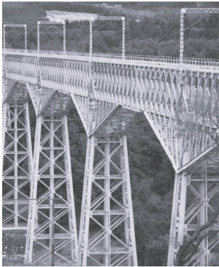
ESTRUCTURA VIADUCTO MALLECO
