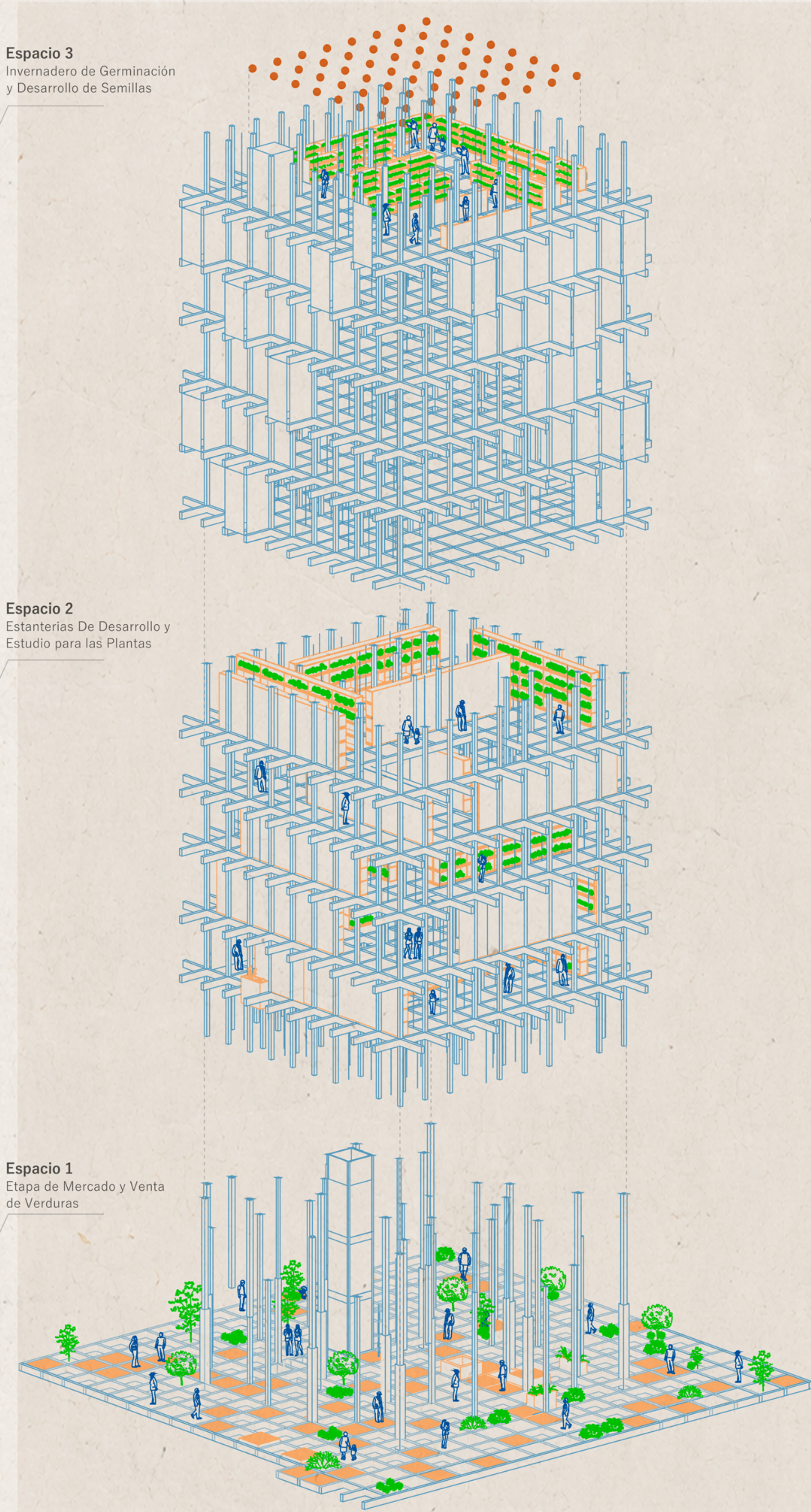
Axonométrica
