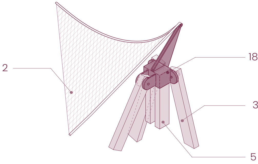
D1. UNIÓN PILAR-CABEZA-TELA
