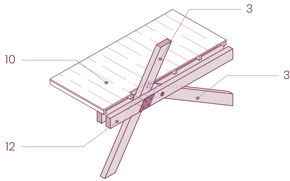
D2. UNIÓN CABALLETE-PLATAFORMA
