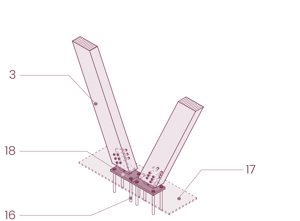
D4. UNIÓN ENTRE CABALLETES
