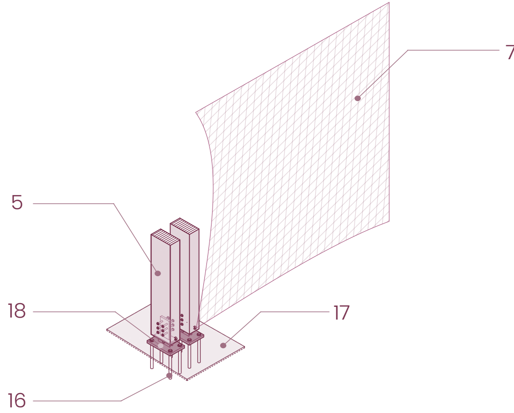
D3. PIE DE PILAR
