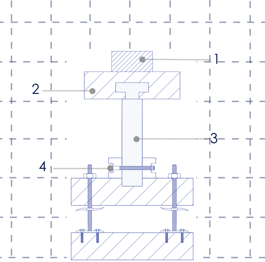
Detalle Riel Esc 1:5
