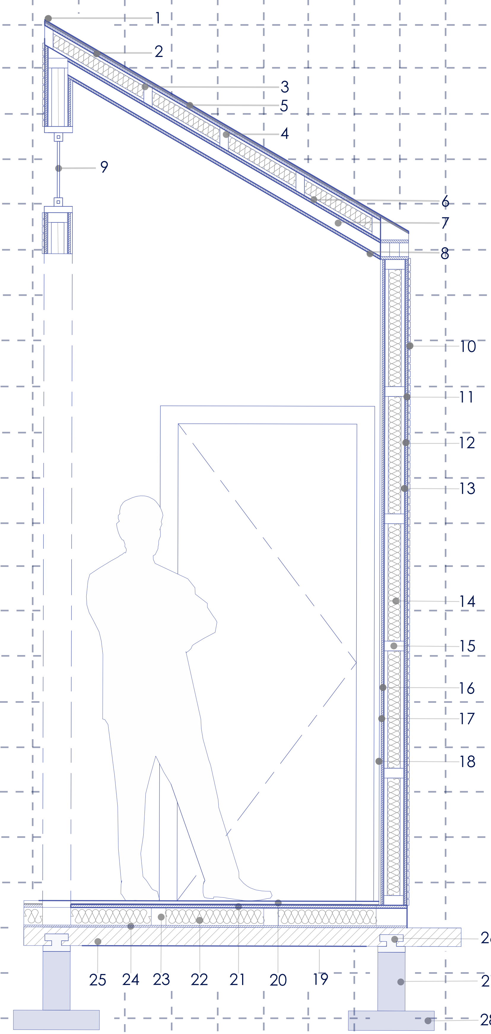
Escantillón Esc 1:10
