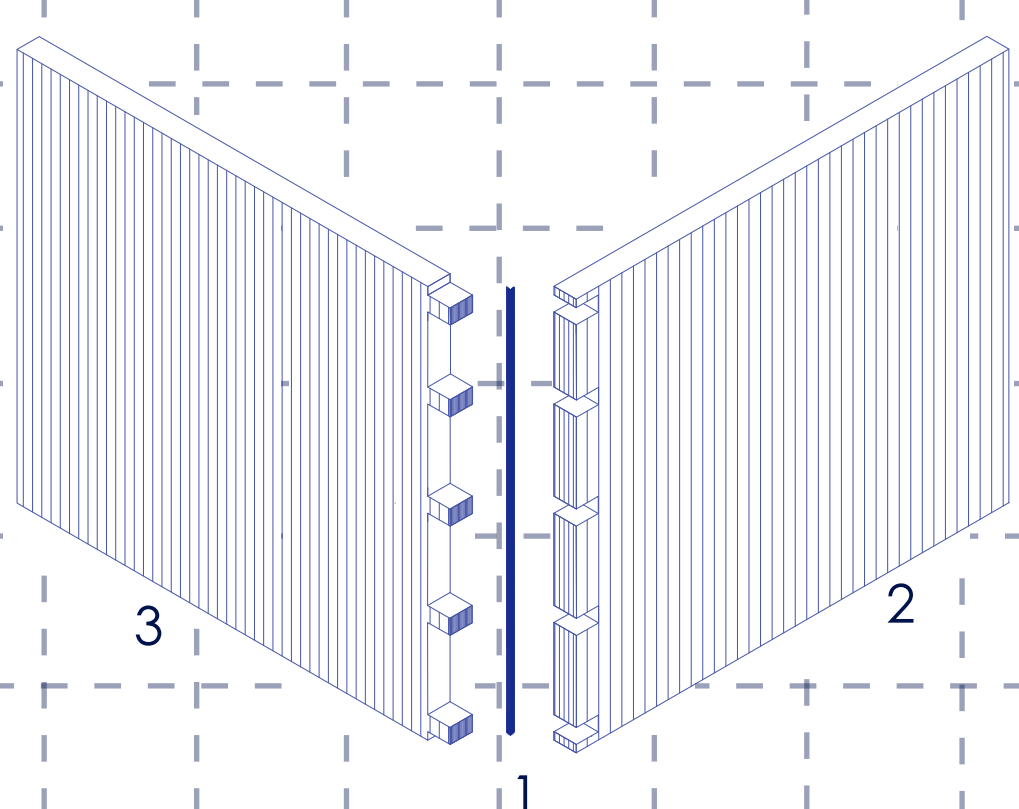
Detalle Unión Muro Esc 1:50
