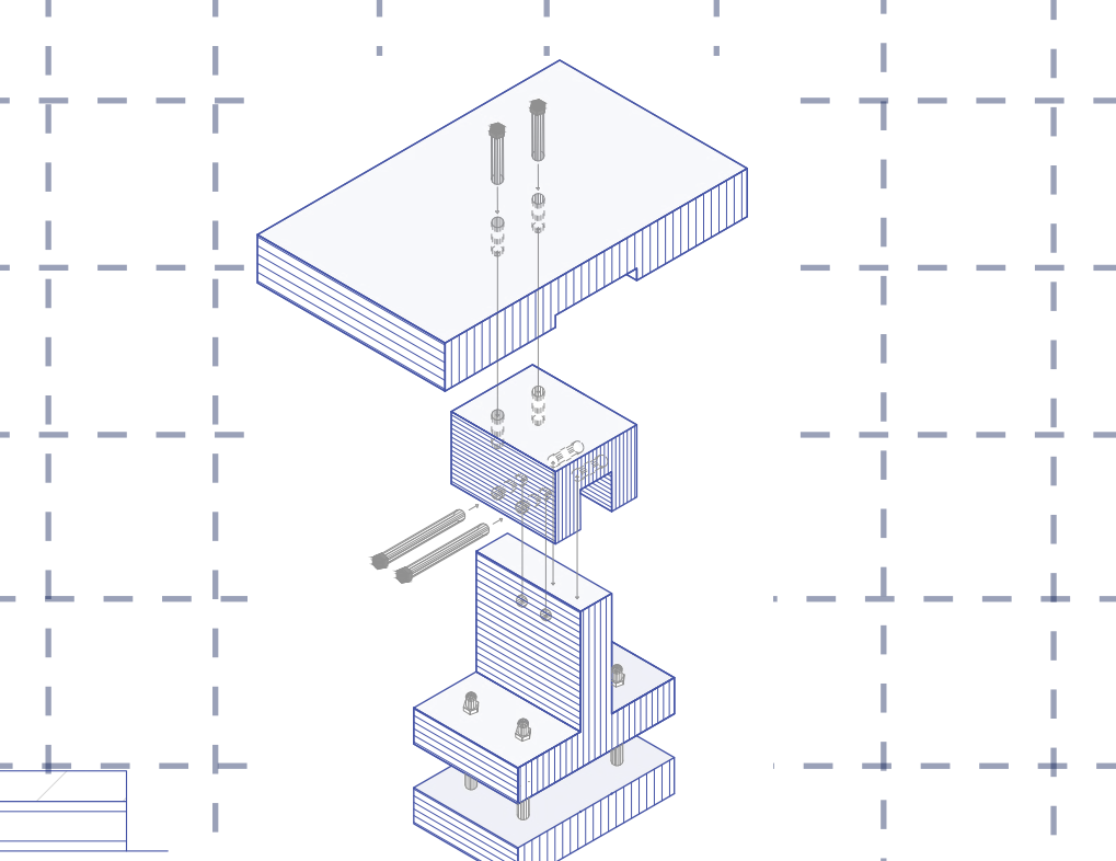
Detalle Riel Explotado Esc 1:10
