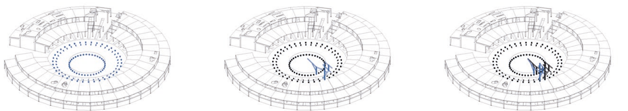
P1 - Trazado y anclaje de columnas P2 - Montaje de módulo constructivo sobre anclajes de columnas P3 - Montaje simétrico radial de módulo constructivo P4 - Unión entre módulos constructivos levantados P5 - Repetición radial de montajes y uniones entre módulos P6 - Coronación con techo entramado prefabricado in-situ
