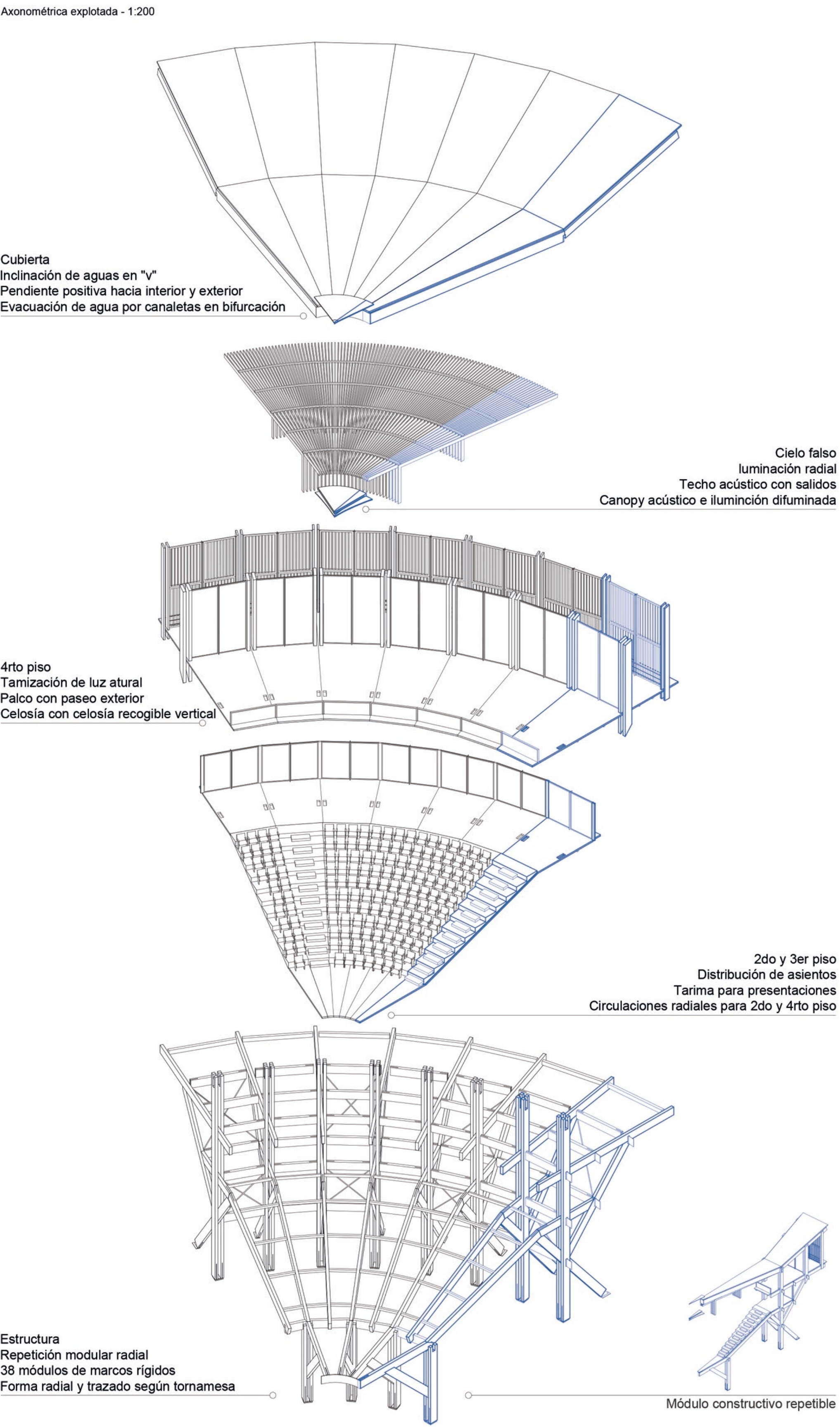
Estructura Repetición modular radial 38 módulos de marcos rígidos Forma radial y trazado según tornamesa
