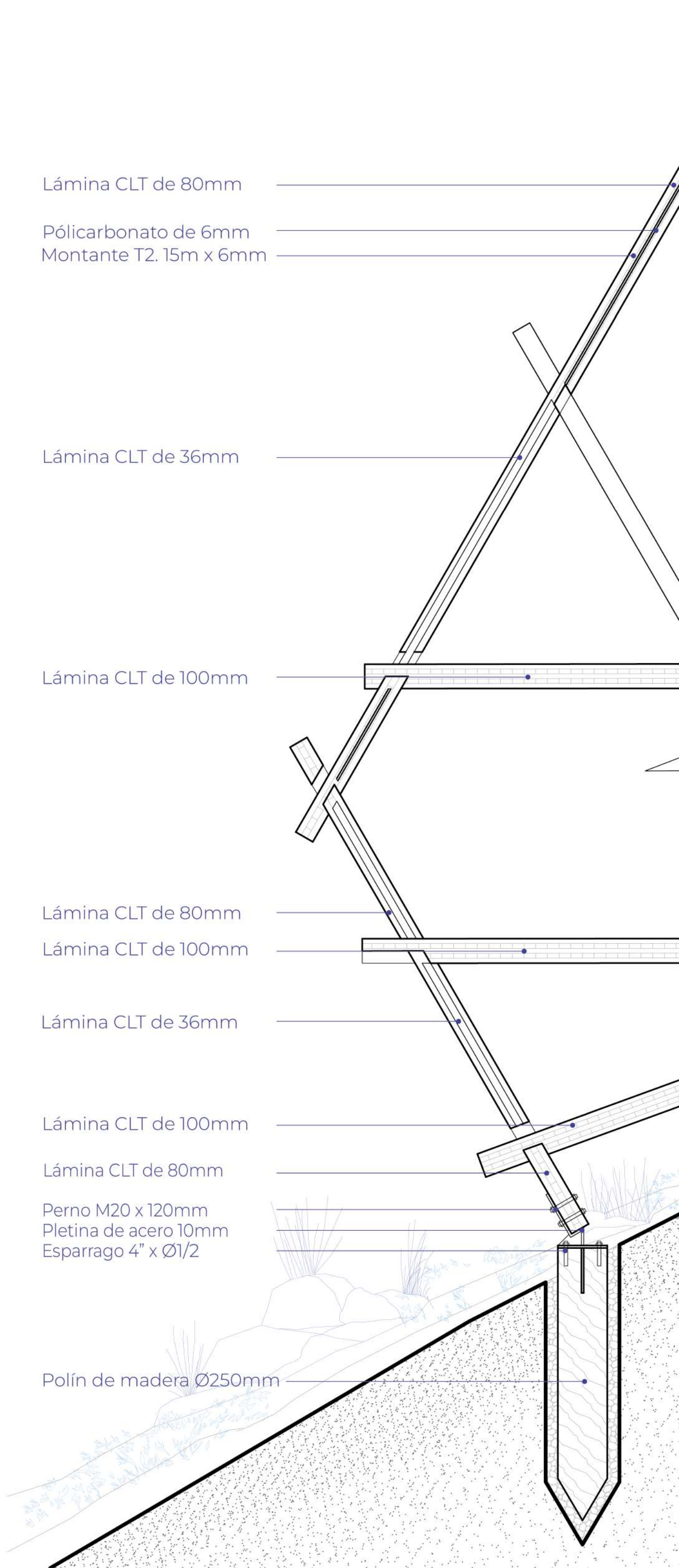
ESCONTILLÓN | ESQ 1:15
