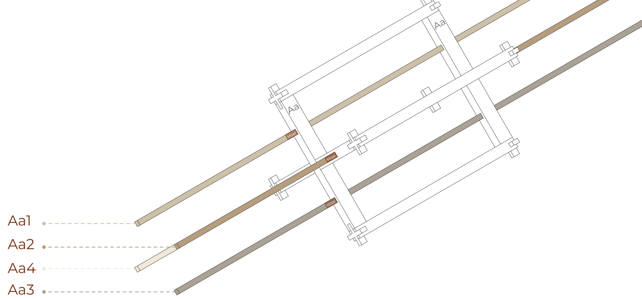
Isométrica funcionamiento grilla Escala 1:100
