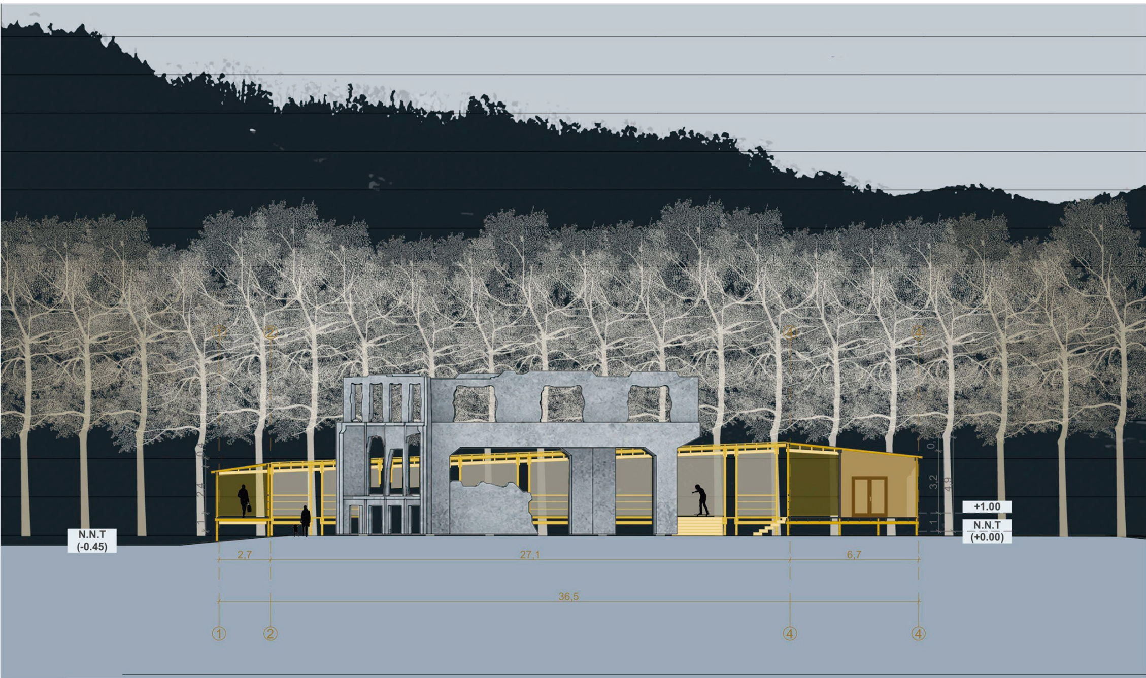
Corte 3 - Escala 1:200
