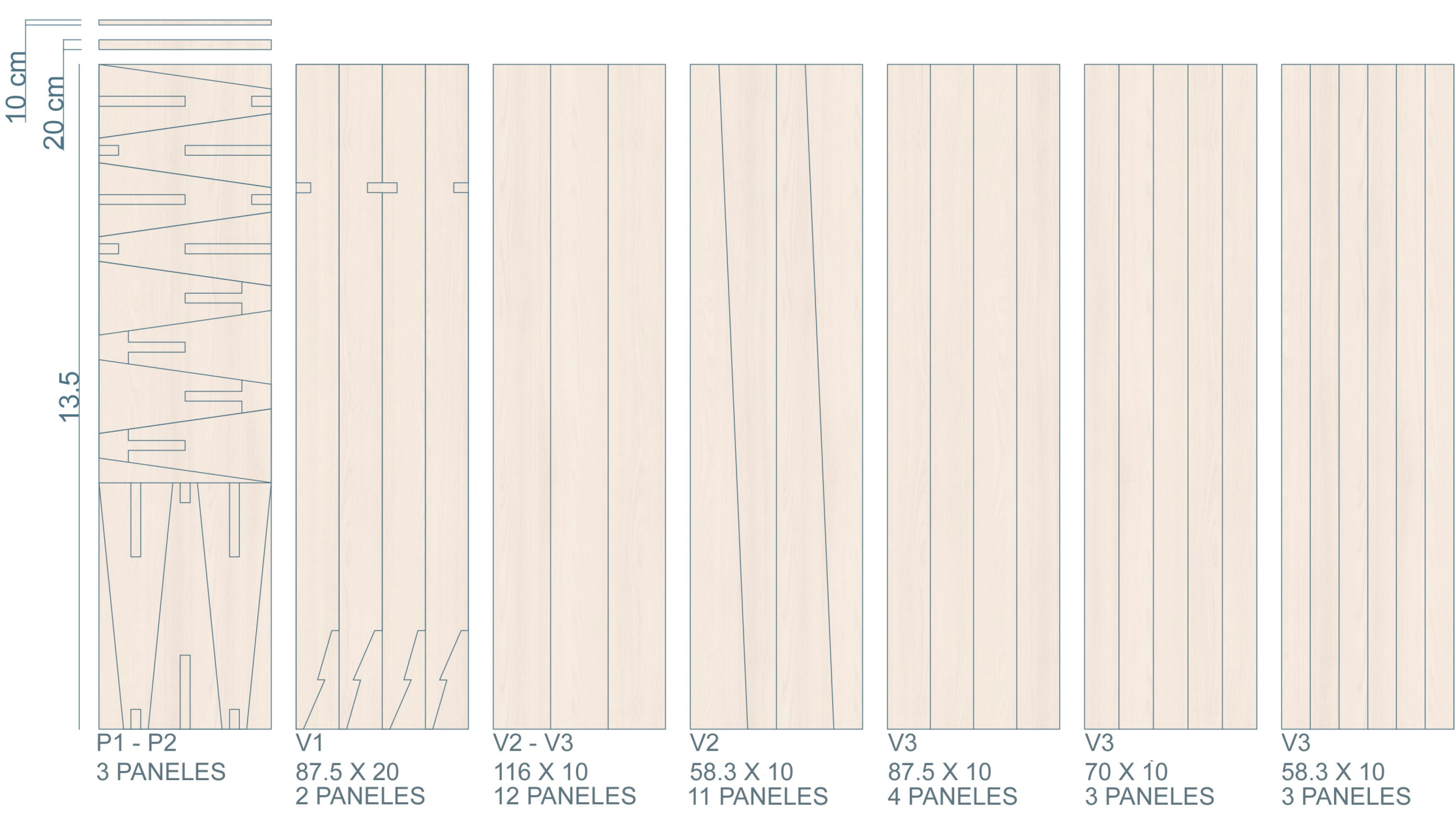
DIMENSIONES - PANEL CLT
