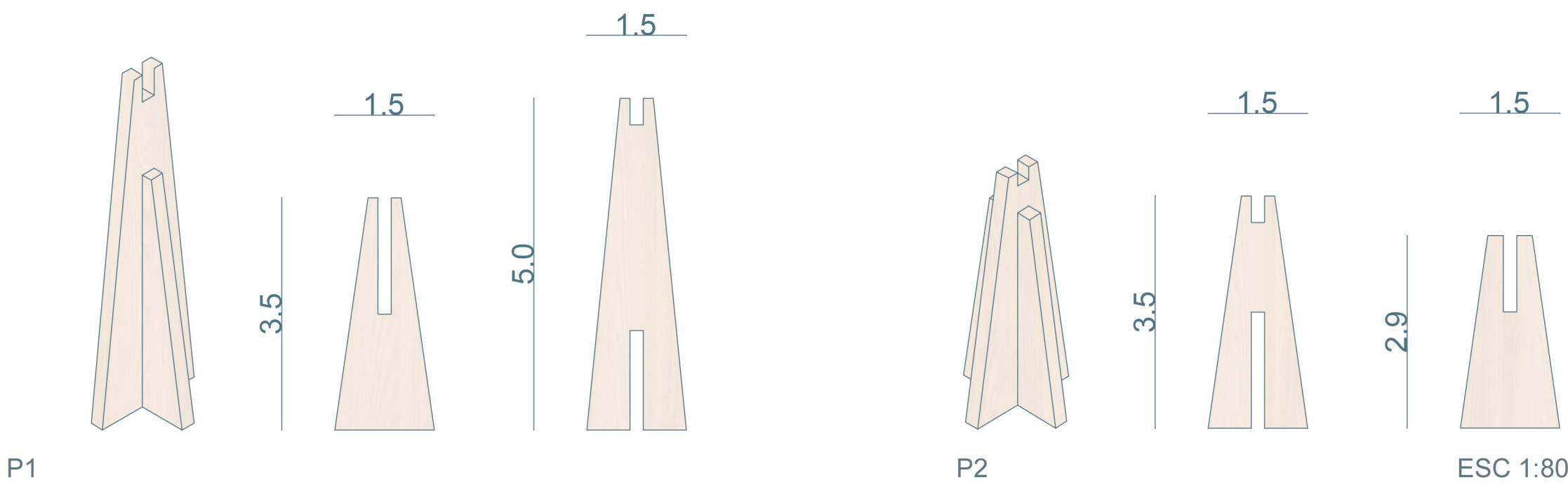
DIMENSIONES - PANEL CLT
