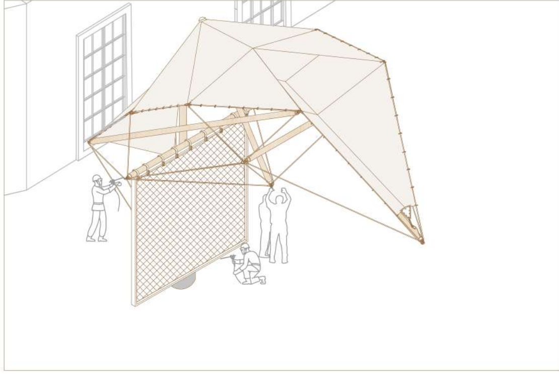
4. Instalación de la Reja
