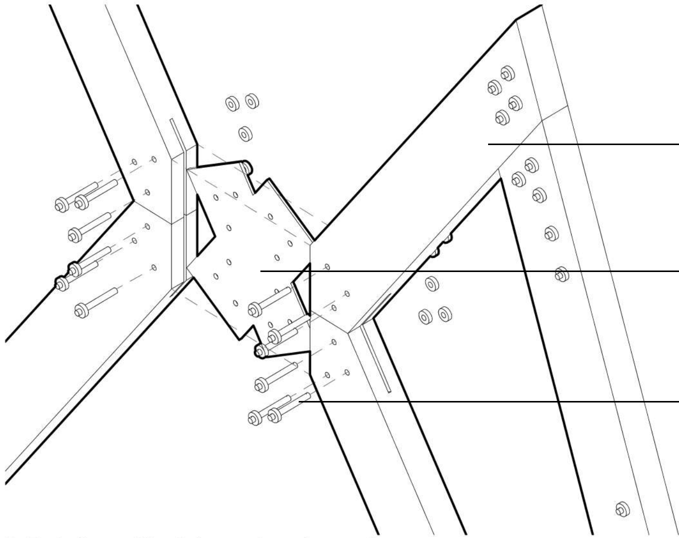
1. Detalle unión triángulos de madera-acero
