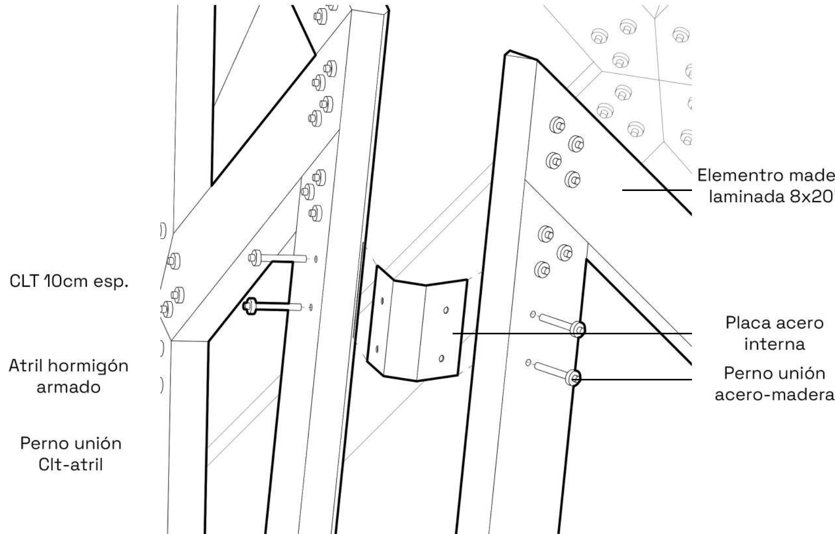
8. Detalle unión caras del módulo
