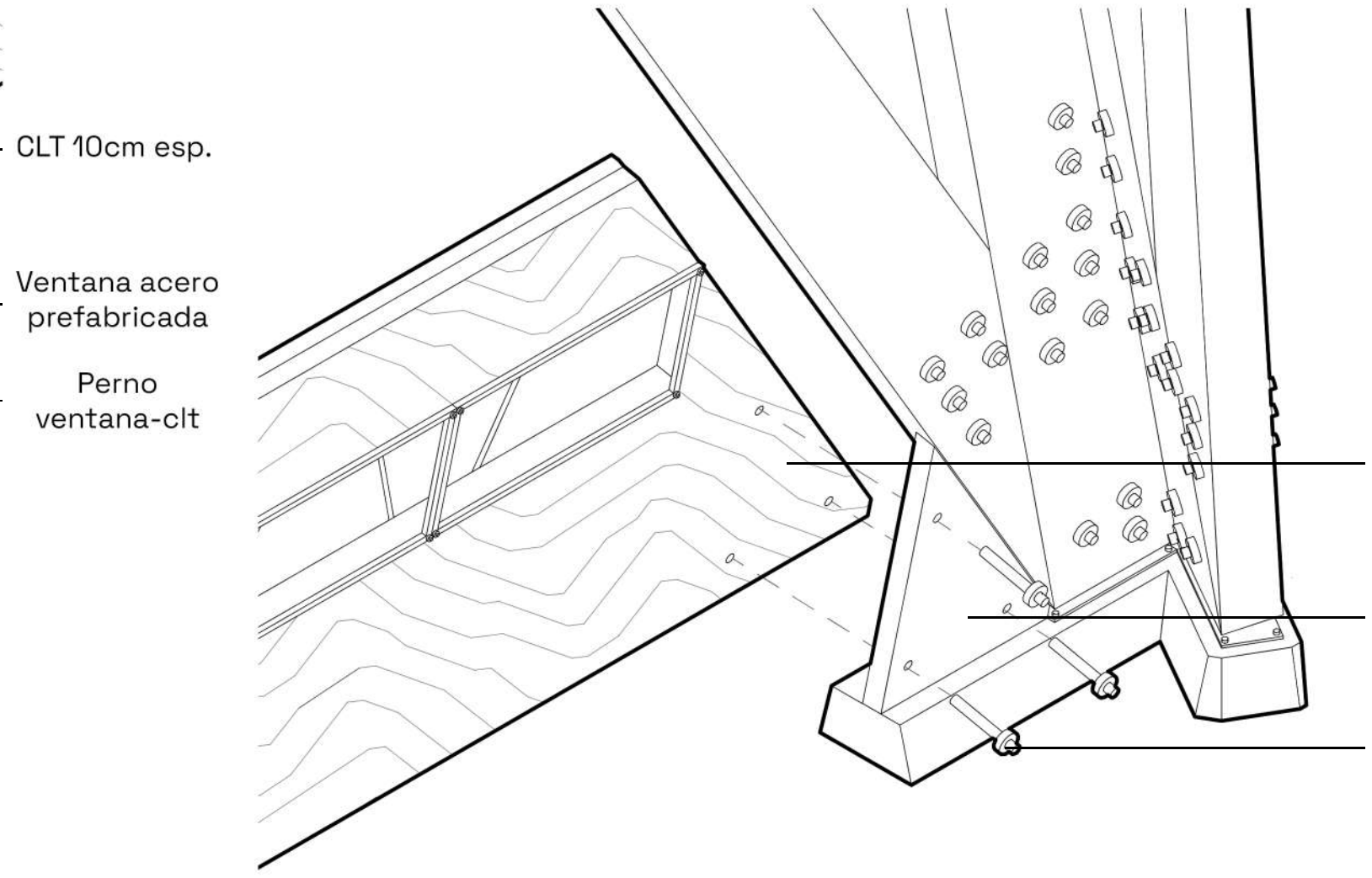
7. Detalle unión CLT-atrial de hormigón
