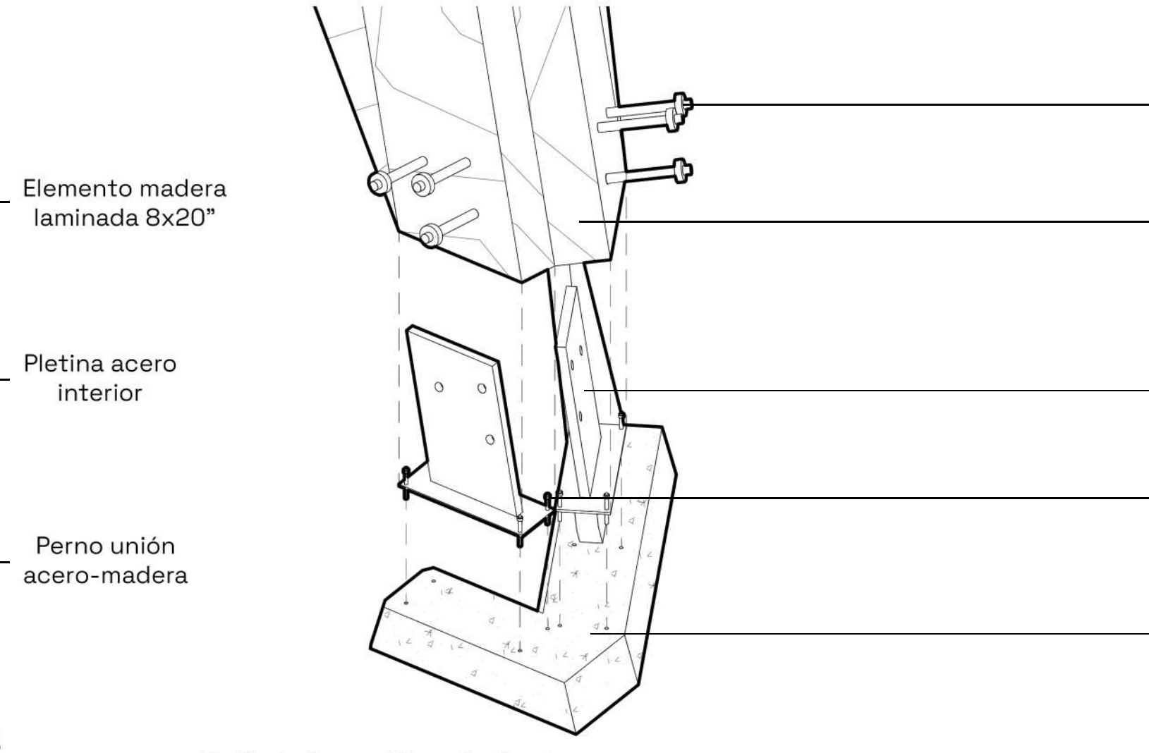
2. Detalle unión cemento
