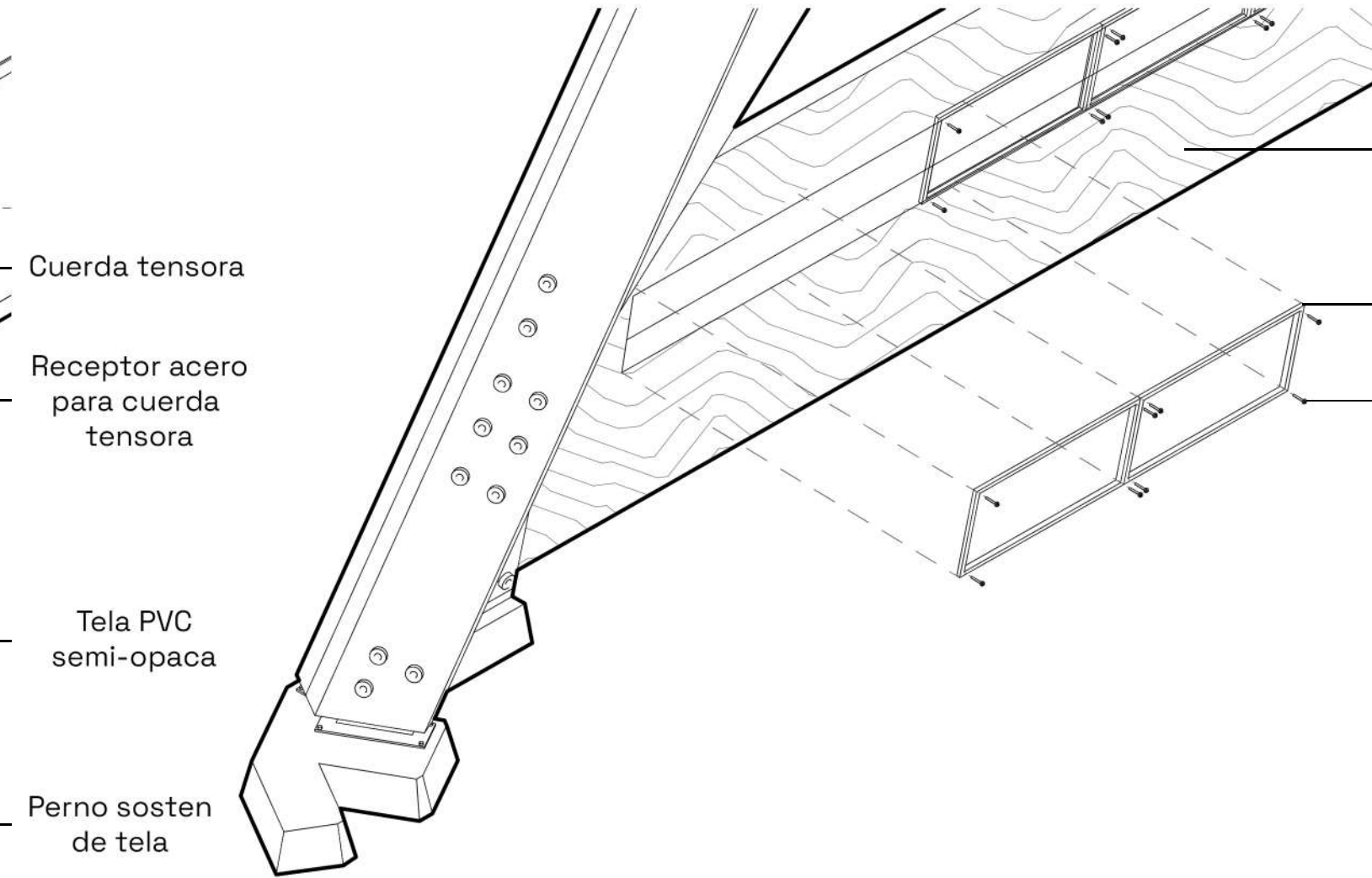
6. Detalle unión ventanas-CLT
