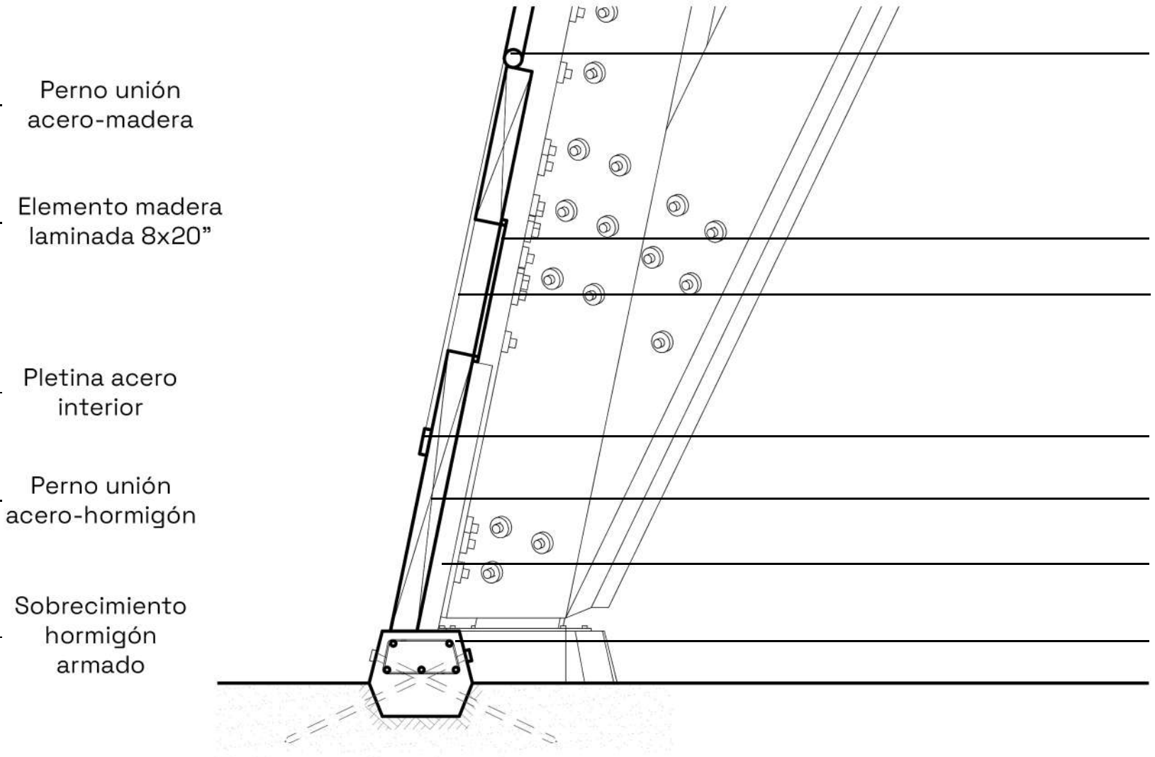
3. Escantillón borde
