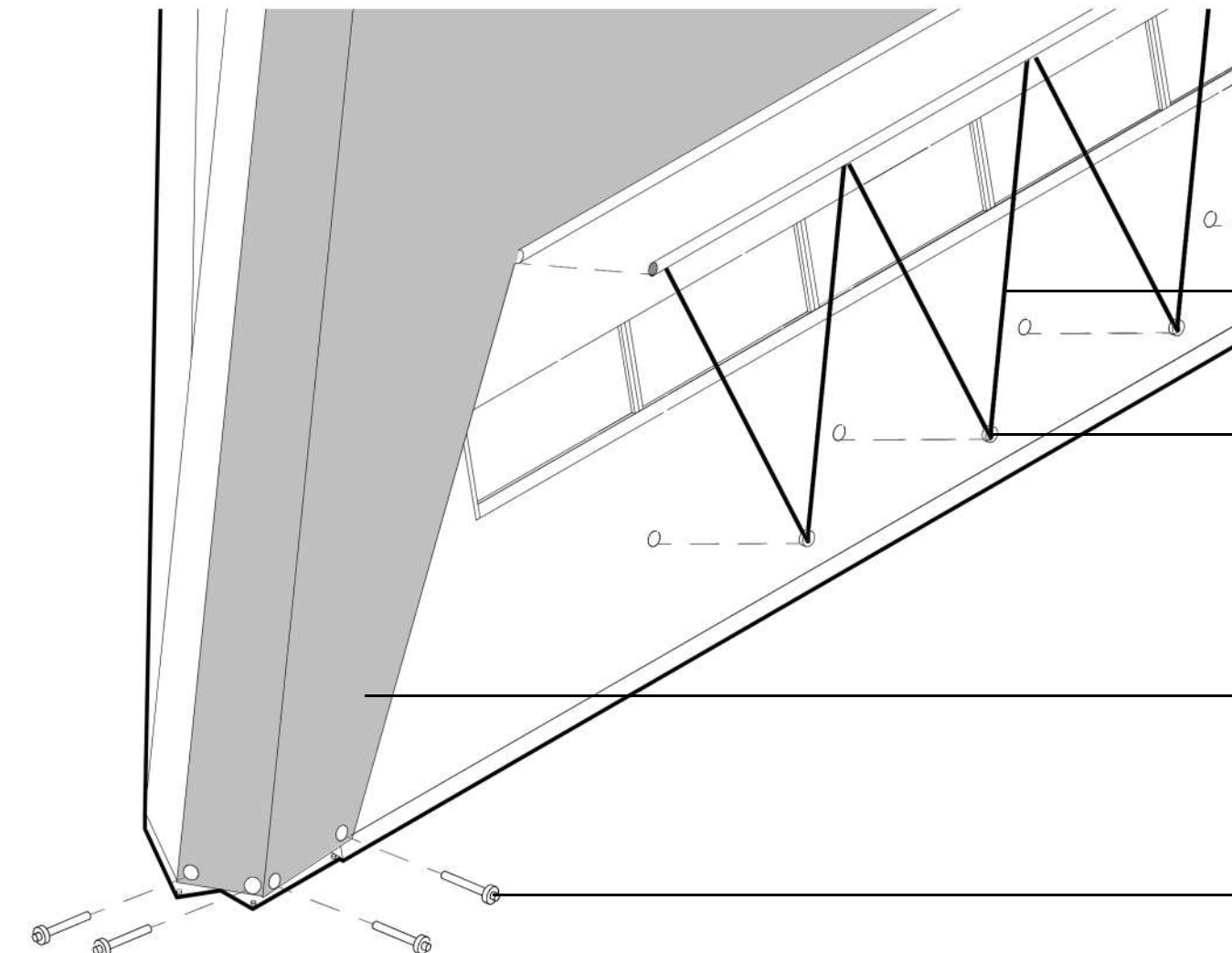
5. Sistema tela y tensado
