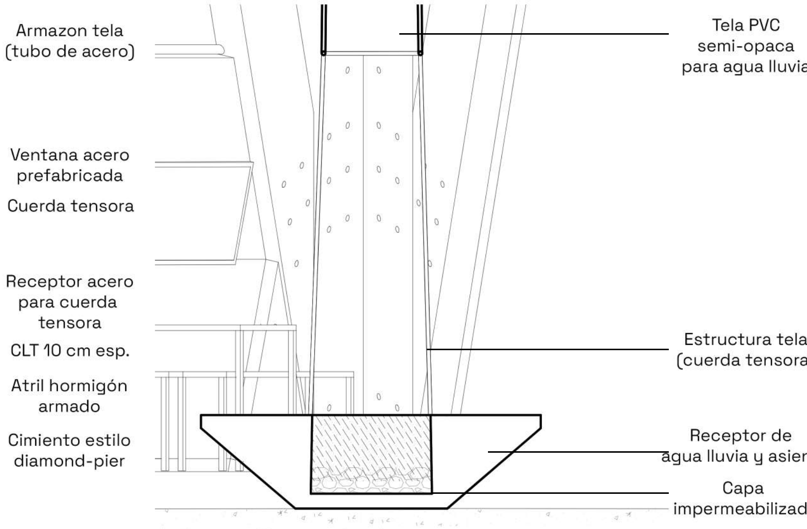
4. Escantillón caída de agua
