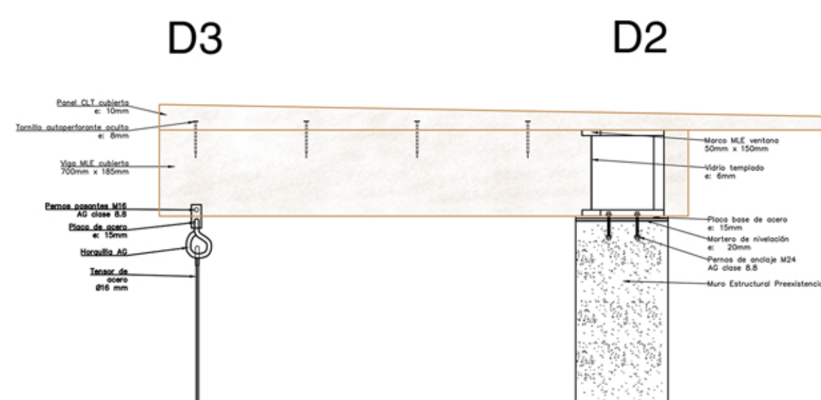
Detalle Techumbre - Muro - Tensor
