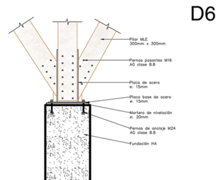
Detalle Hormigón - Pilar
