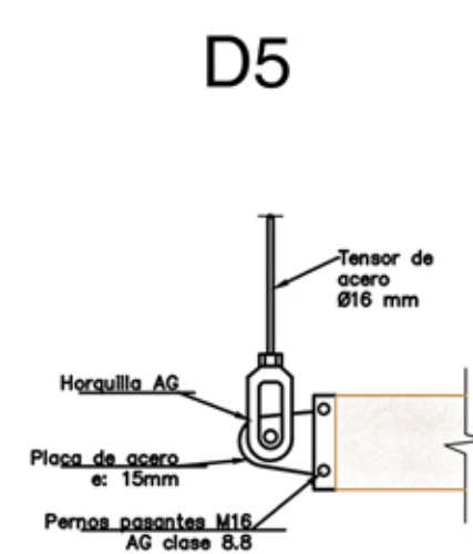
Detalle Rampa - Tensor
