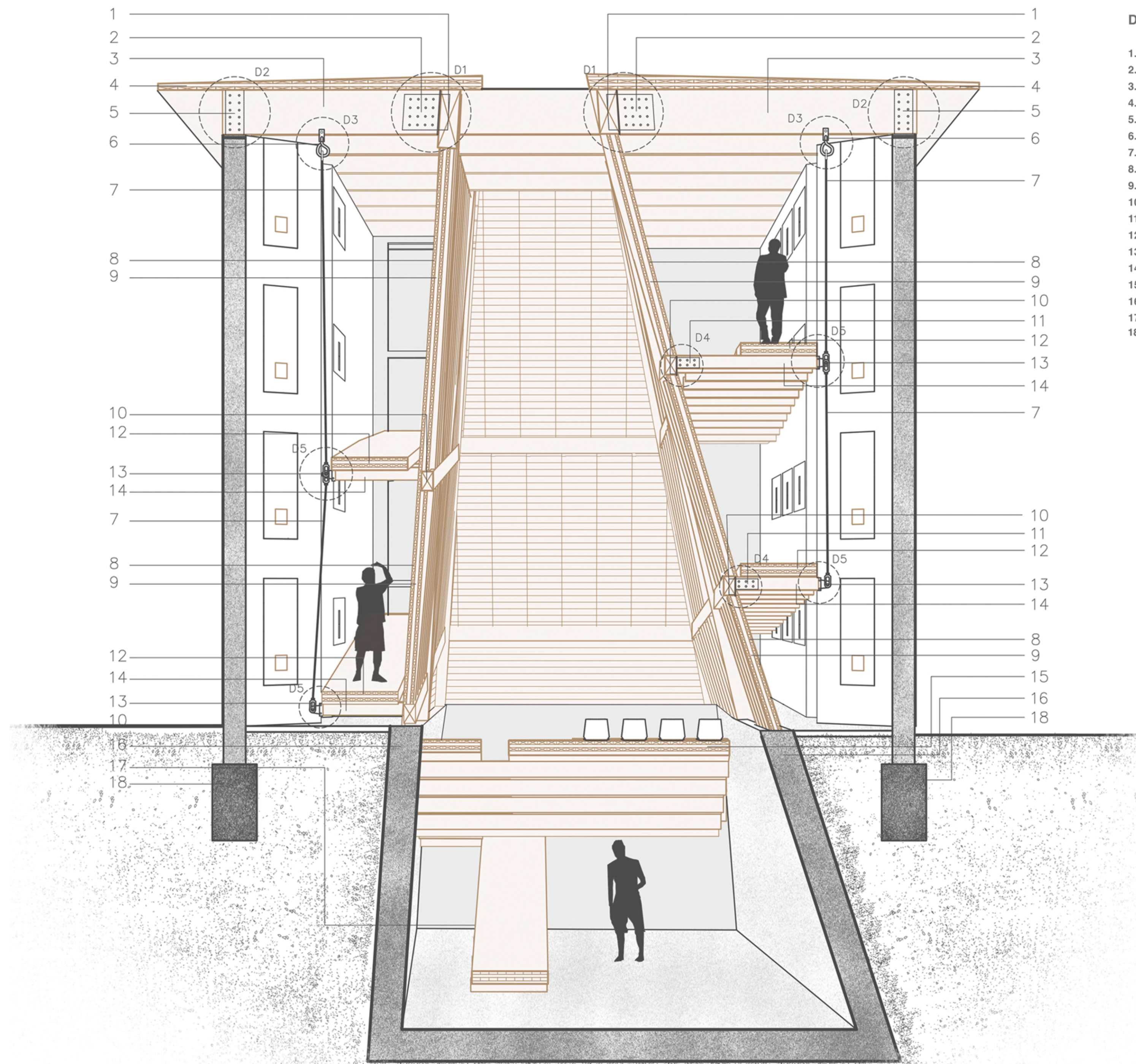
Corte Escantillón Esc 1:50
