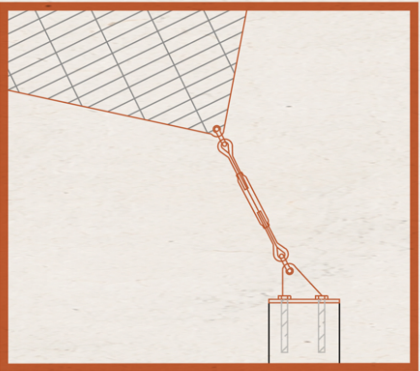
Unión de la lona mediante tensor
