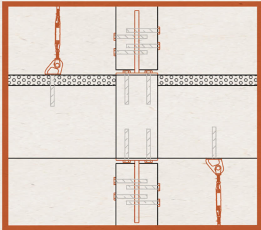
Vínculo de tensores y placas de acero a las vigas de madera
