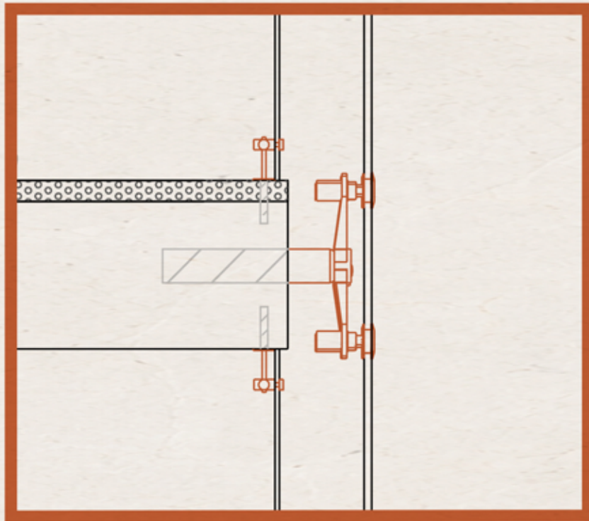
Anclaje de los dilatadores de aluminio a las vigas de madera
