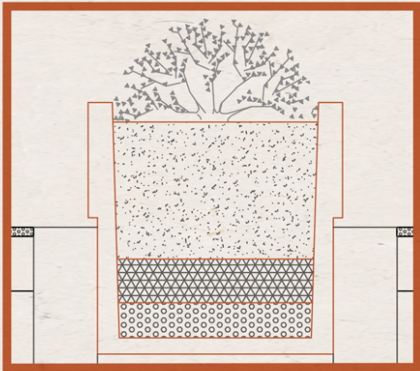
Estructura interna de los maceteros
