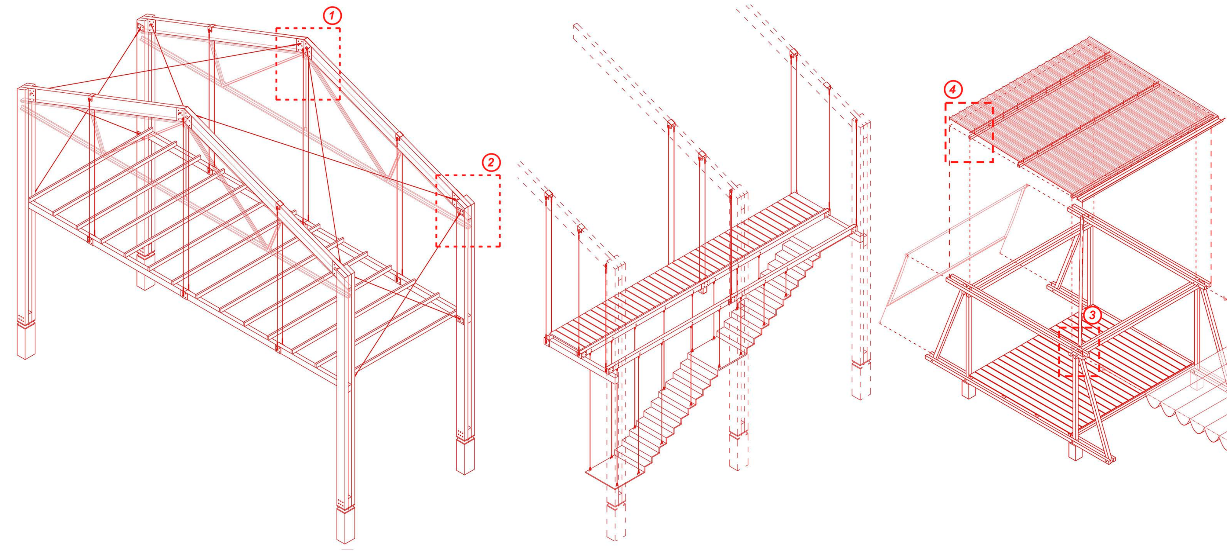
SISTEMA ESTRUCTURAL. MÓDULOS ESTRUCTURALES + DETALLE DE UNIONES Y ENCUENTROS.
