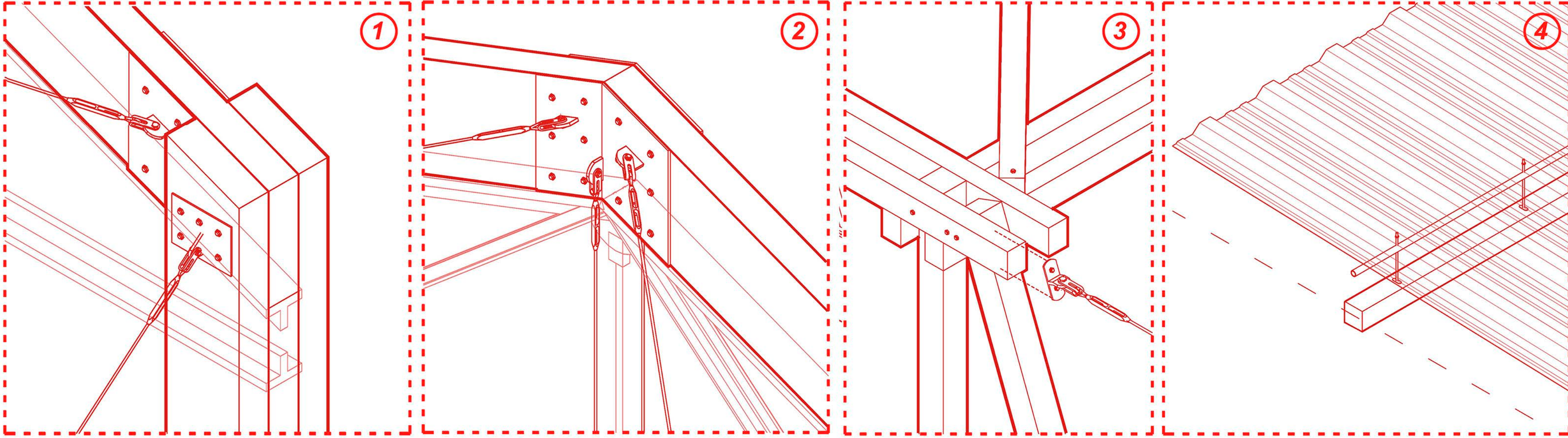
SISTEMA ESTRUCTURAL. MÓDULOS ESTRUCTURALES + DETALLE DE UNIONES Y ENCUENTROS.
