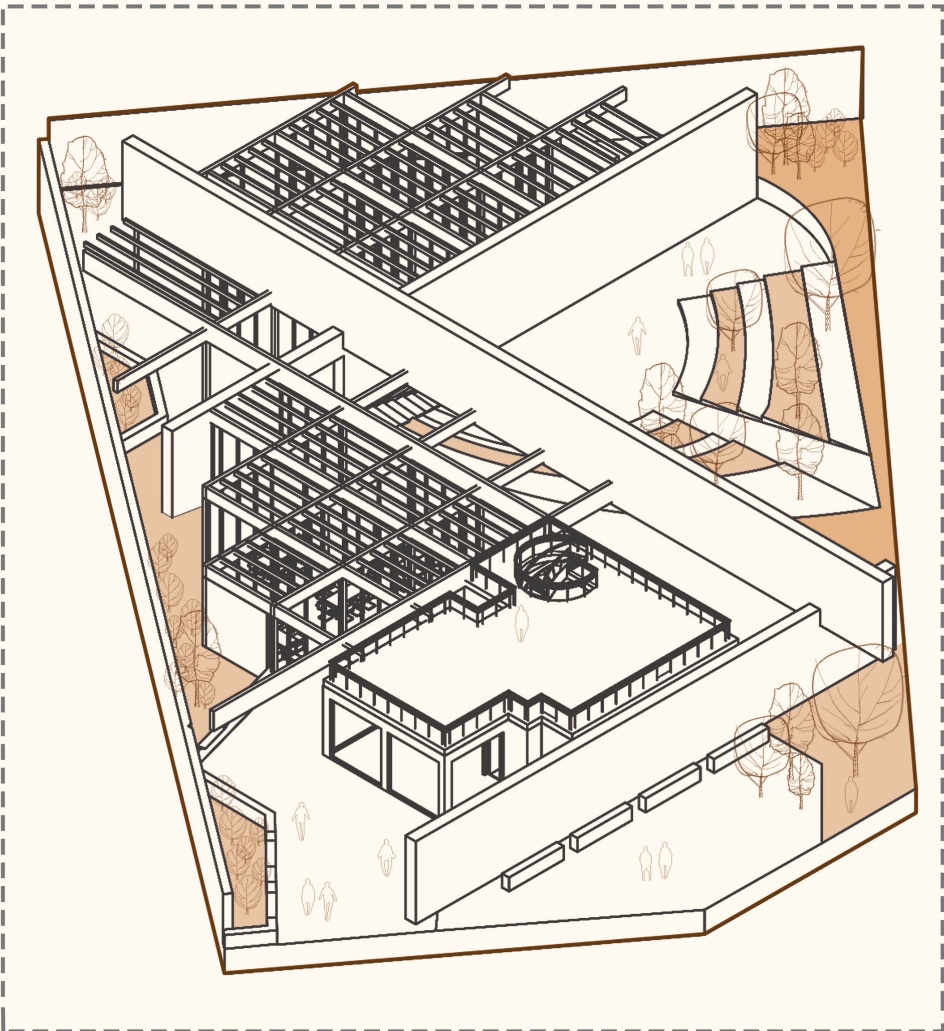
Isometrica
