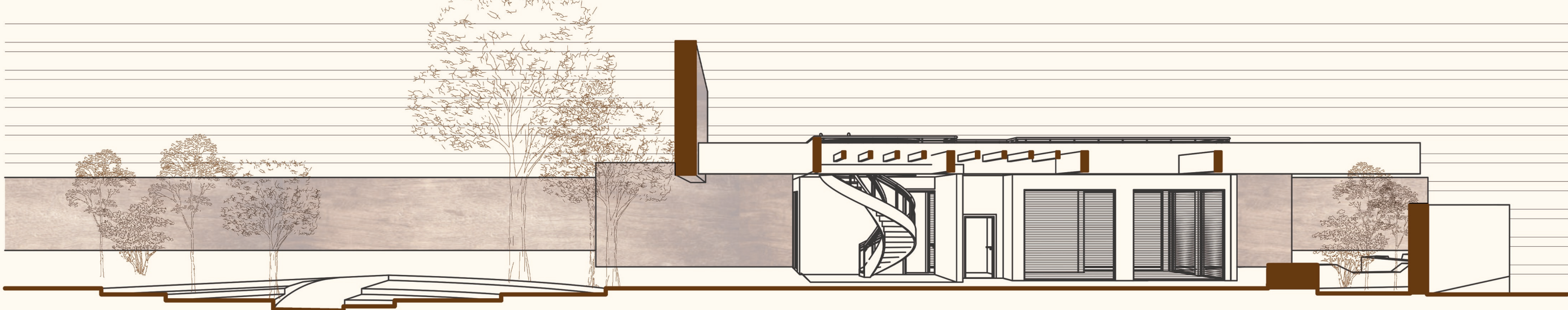
Corte C-C' Esc. 1:200
