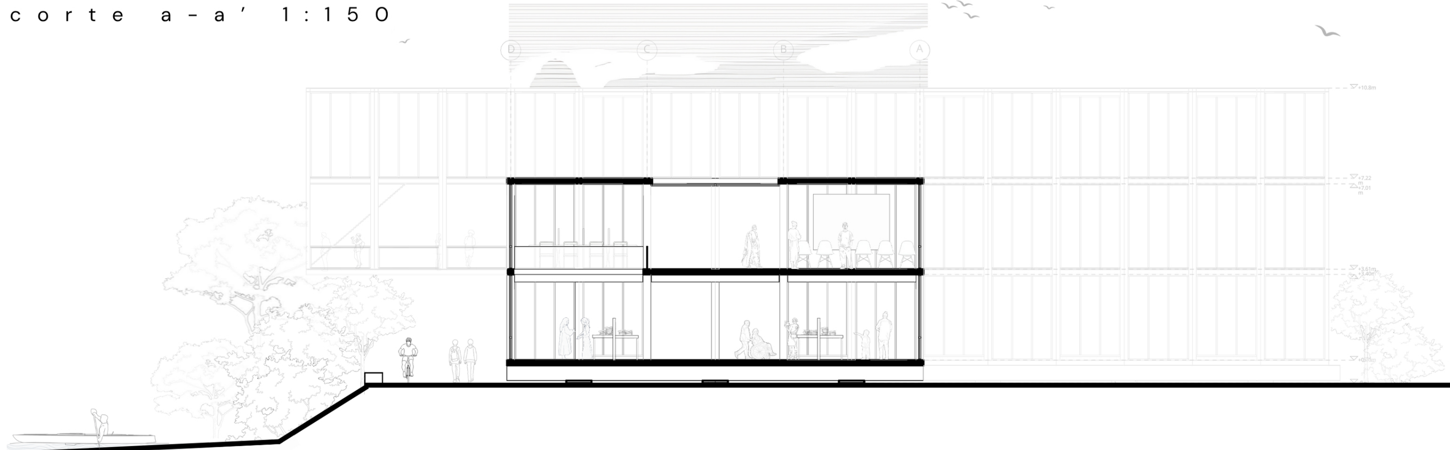
corte a-a' 1:150
