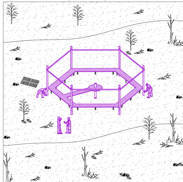
ETAPA 2: PILARES Y PLATAFORMA
