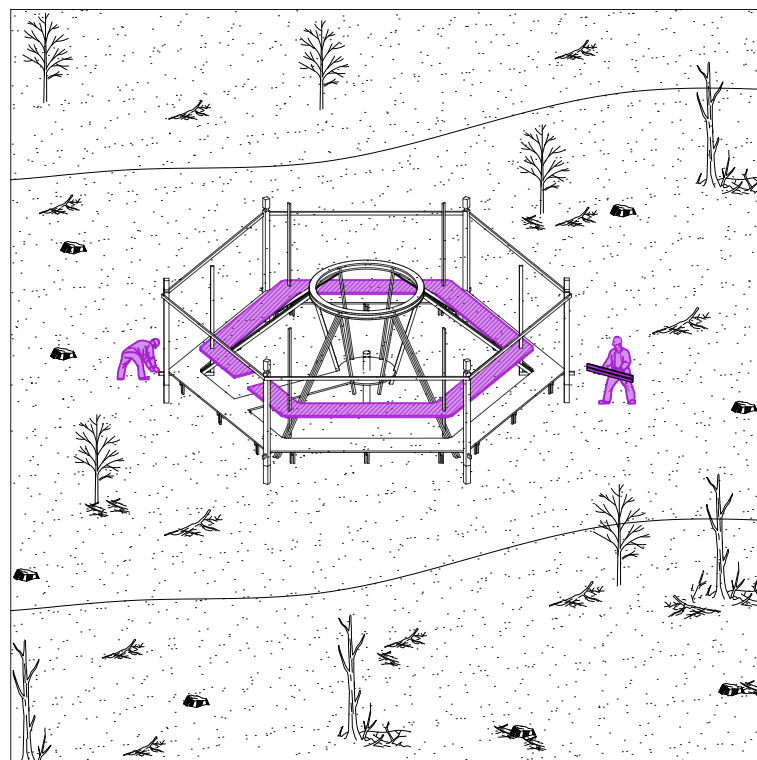
ETAPA 4: MESÓN DE TRABAJO
