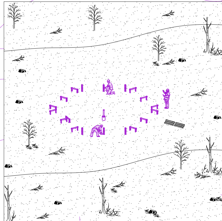
ETAPA 1: SOPORTES Y FUNDACIONES
