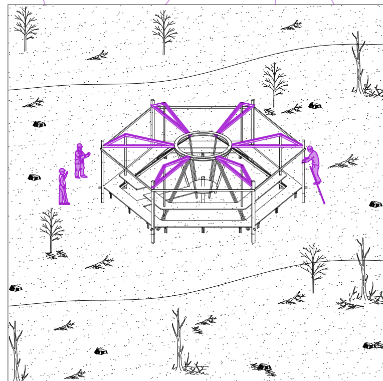
ETAPA 5: CERCHAS ESTRUCTURALES
