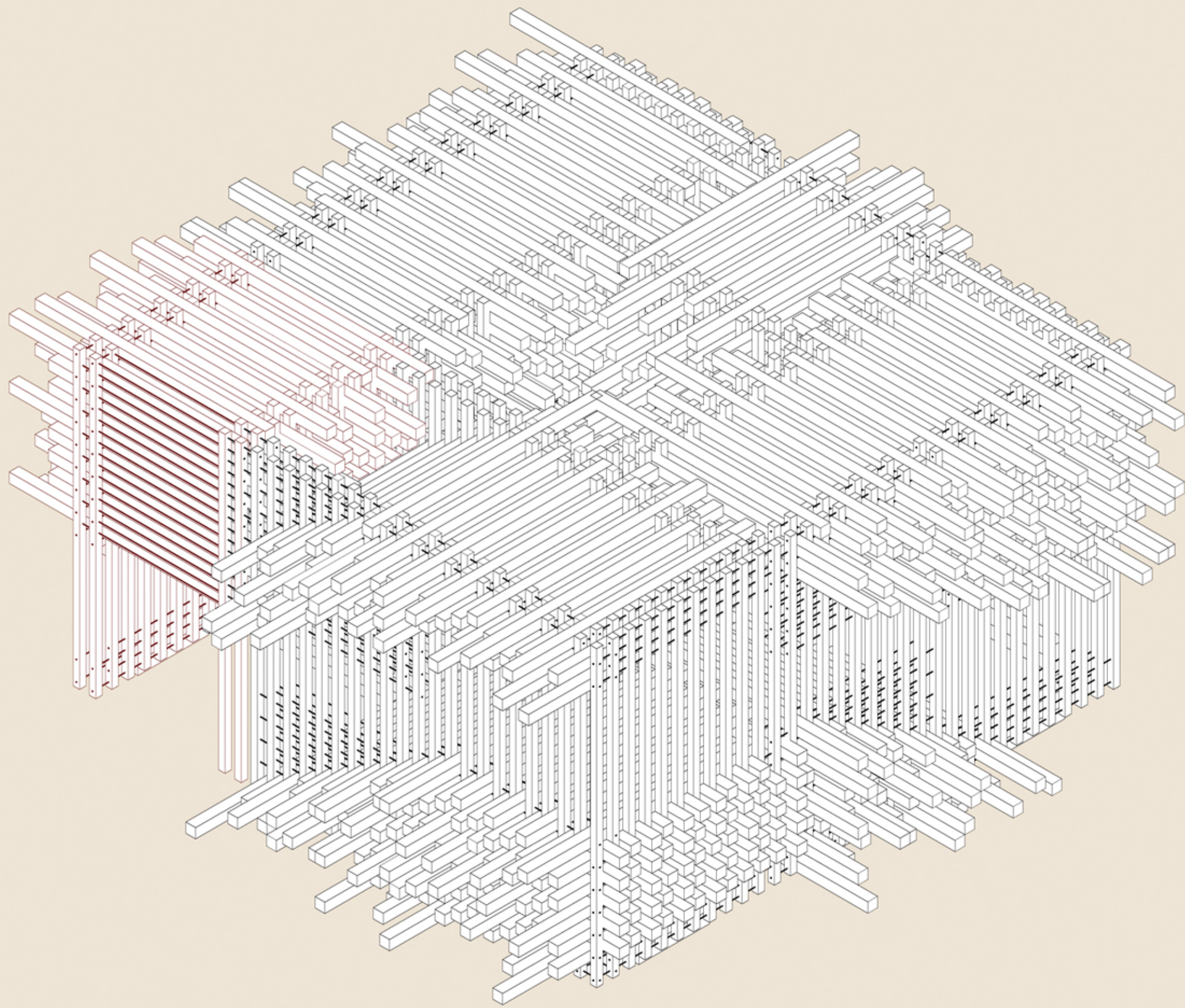
Isométrica de montaje
