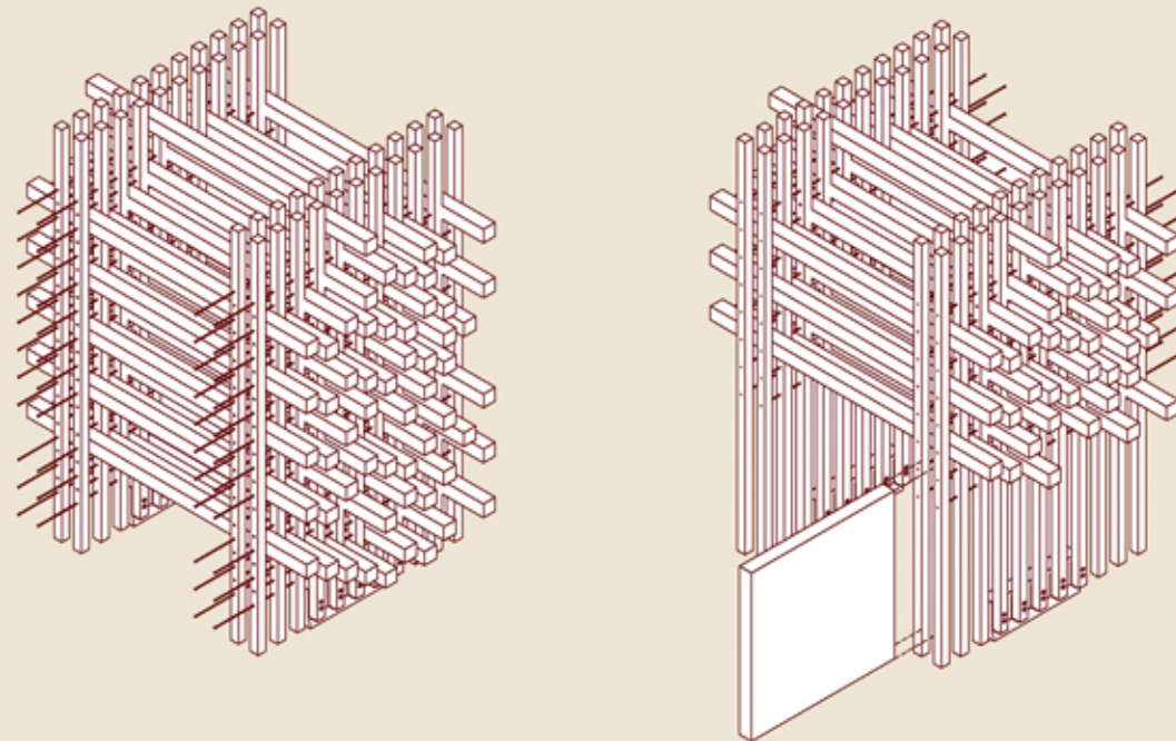
Paso 5t. Esc. 1/75
