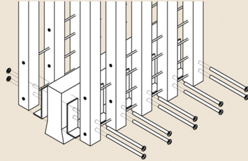
Detalle 1. Esc. 1/20
