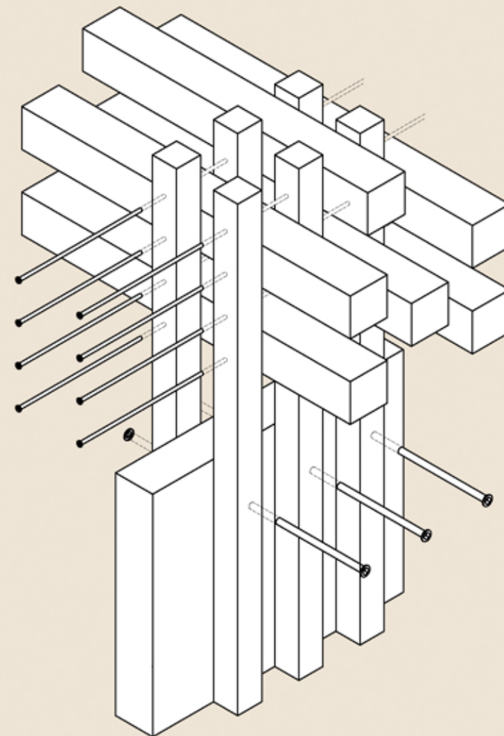
Detalle 3. Esc. 1/20
