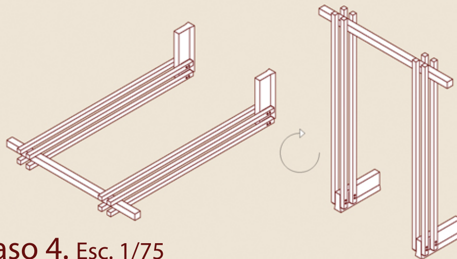
Paso 4. Esc. 1/75
