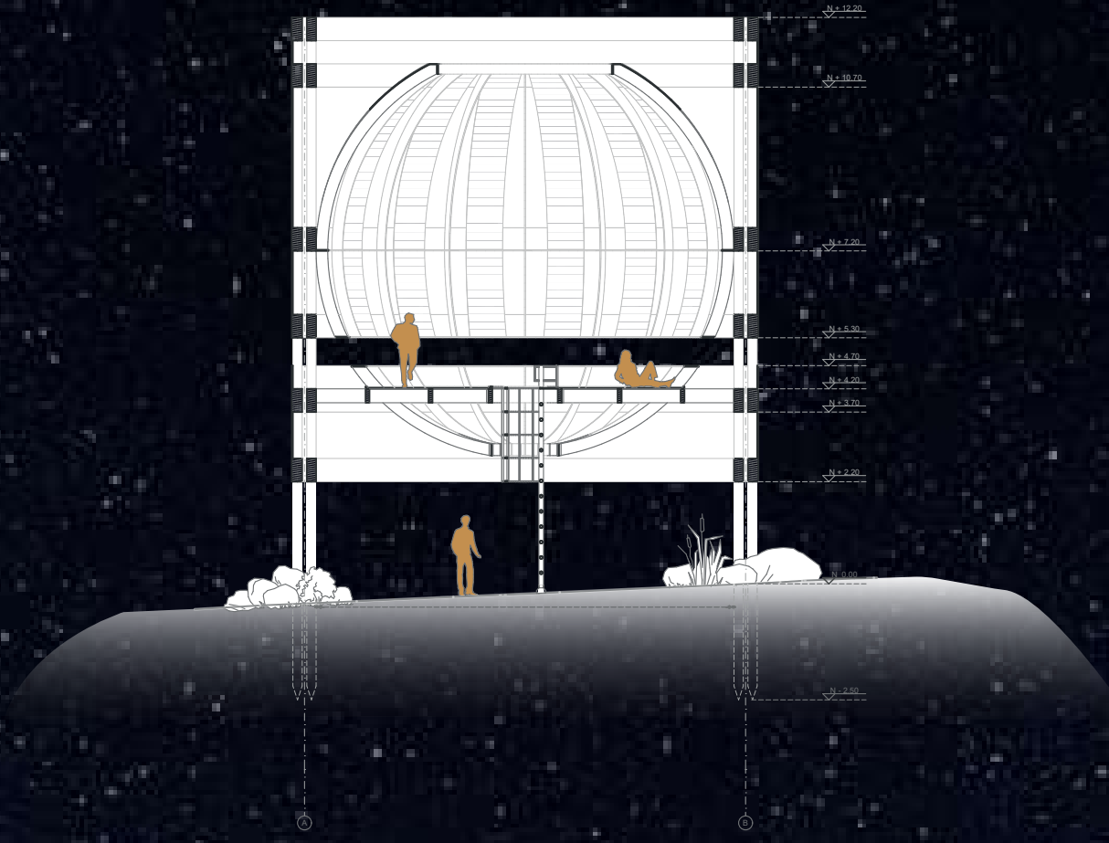
CORTE A-A'
