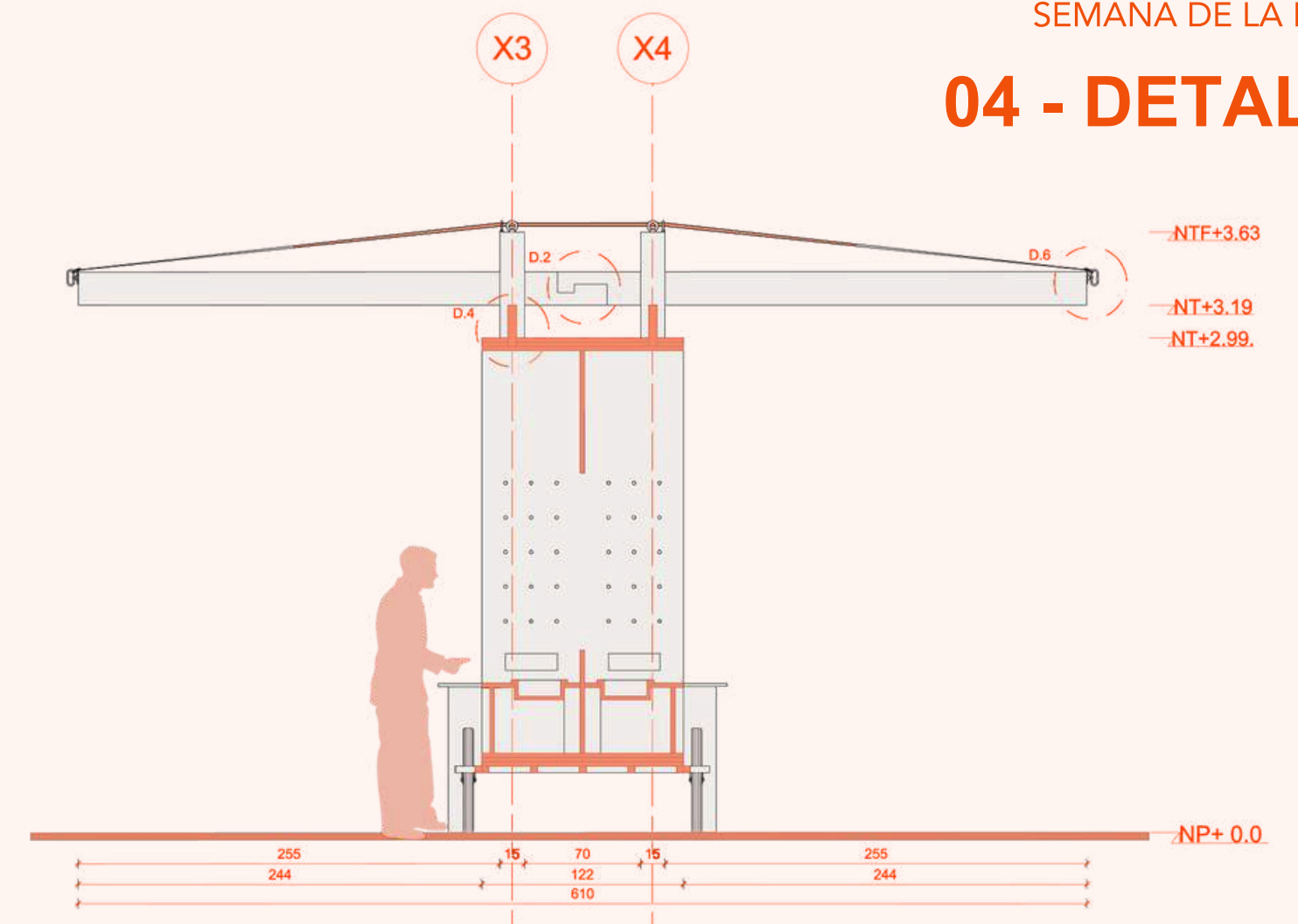
CORTE TRANSVERSAL B'B ESC 1/40
