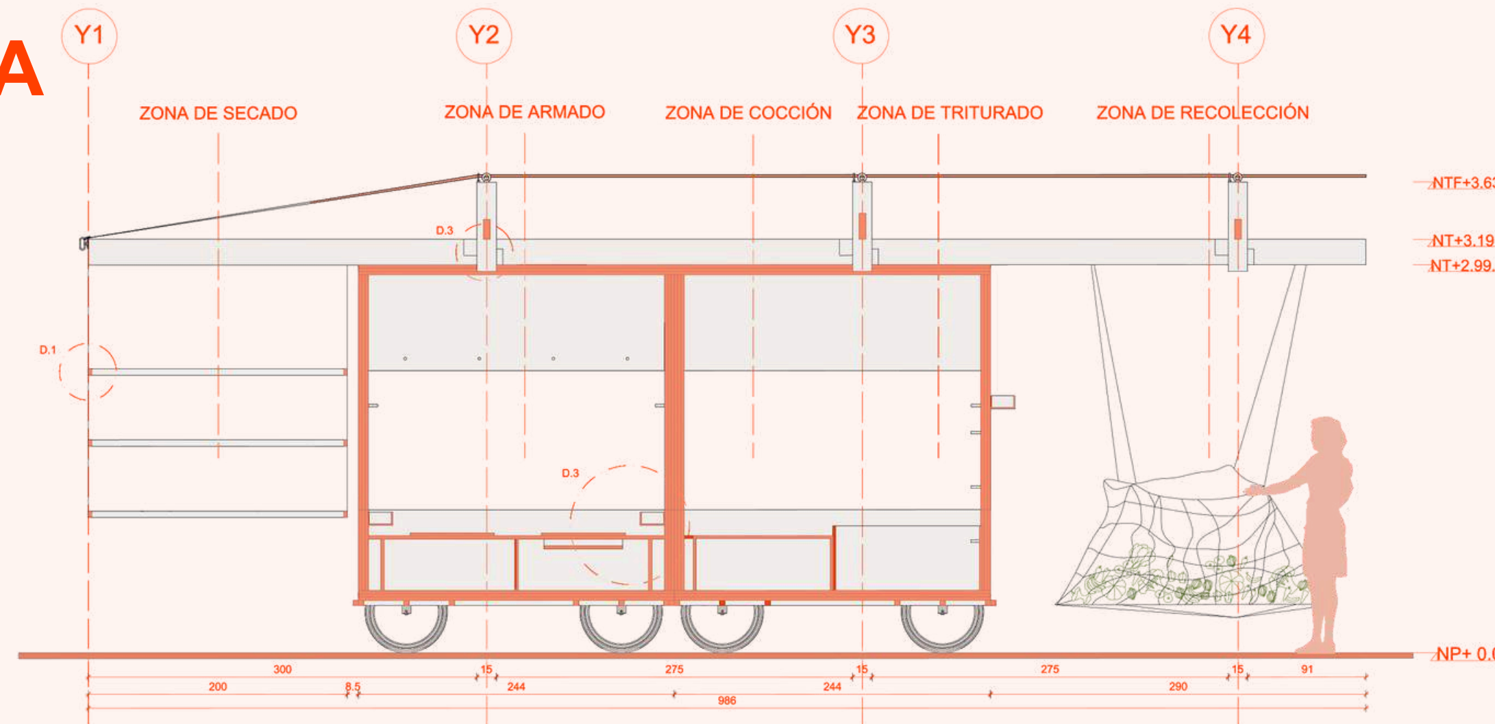
CORTE LONGITUDINAL A'A ESC 1/40
