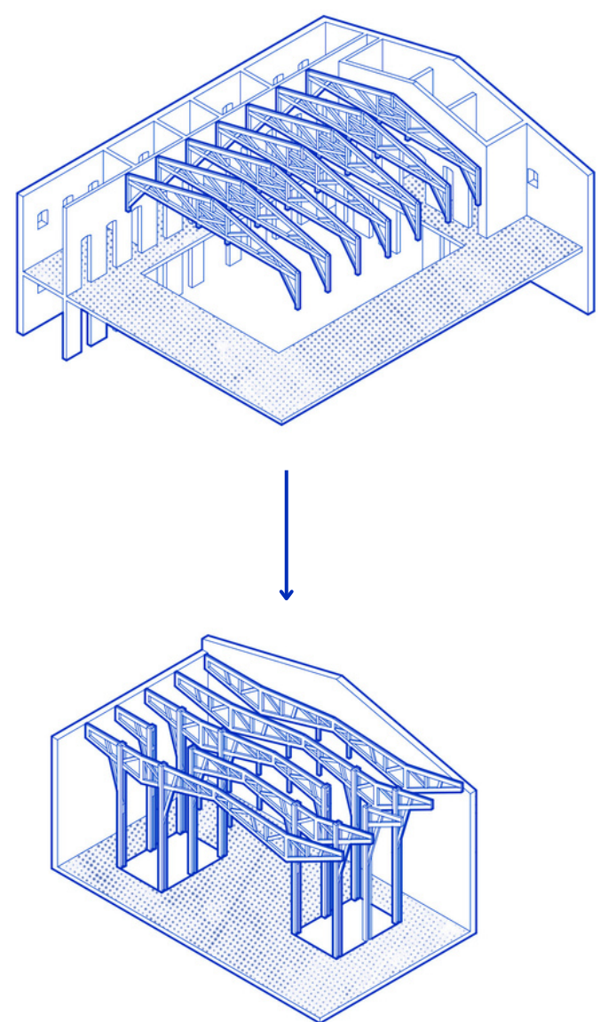
ESQUEMA DE REINTERPRETACIÓN - CERCHA
