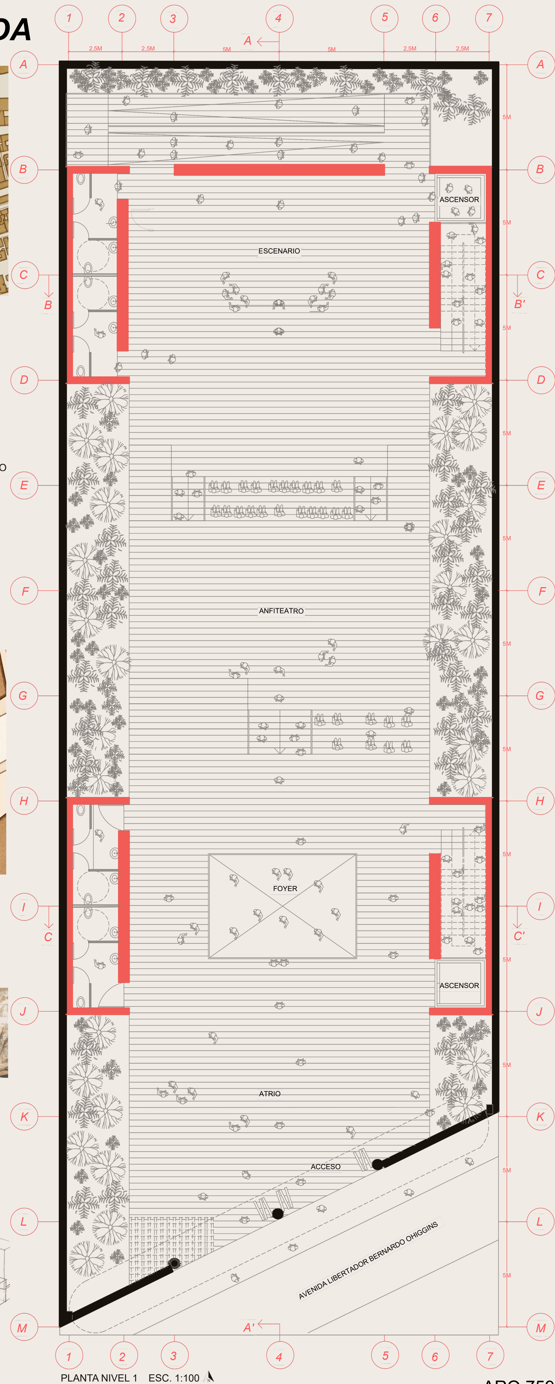
PLANTA NIVEL 1 ESC. 1:100
