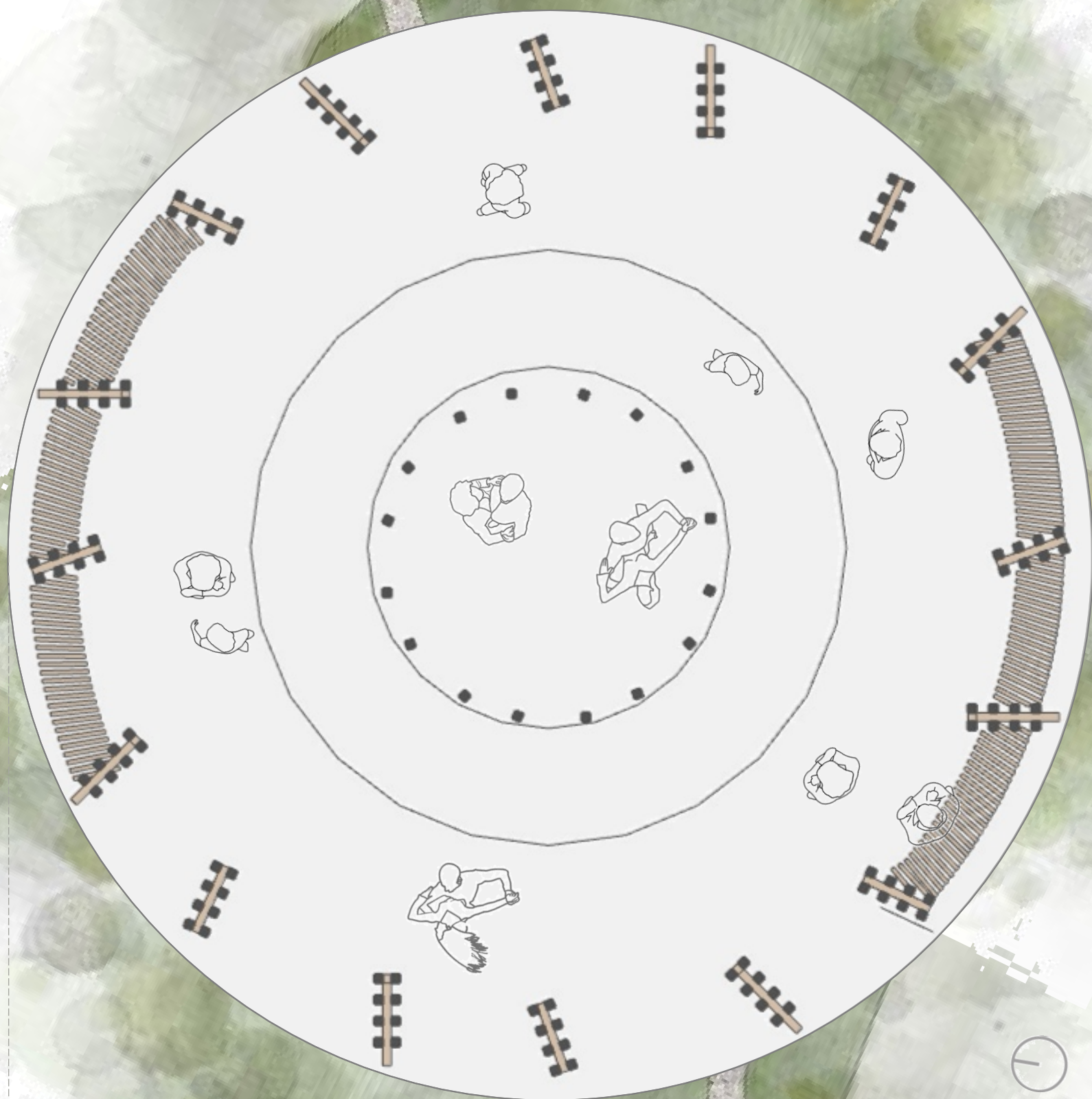
PLANTA SUM
