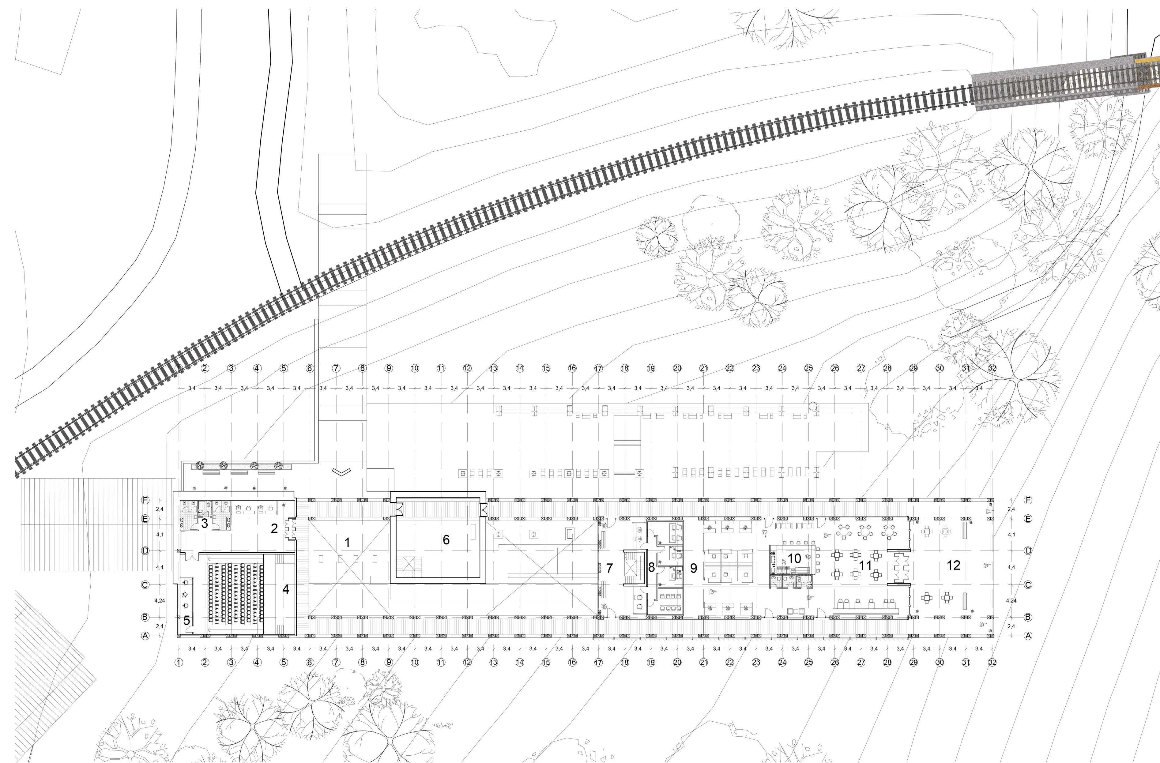
PLANTA ARQUITECTURA PRIMER NIVEL
