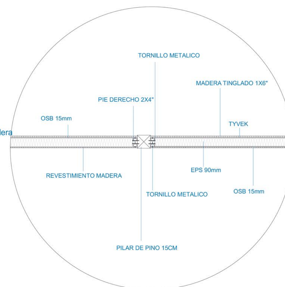
PLANTA PANEL SIP + ESTRUCTURA MADERA
