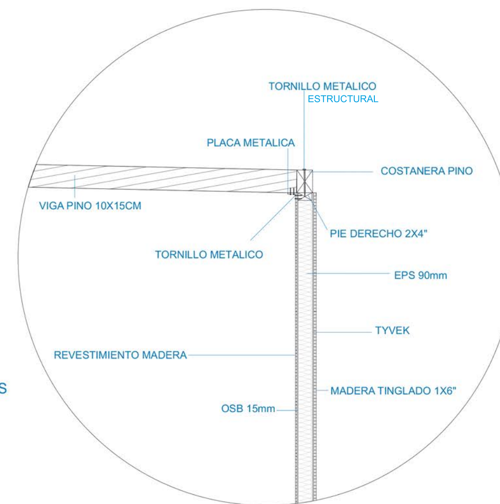
VIGA-PILAR-MURO
