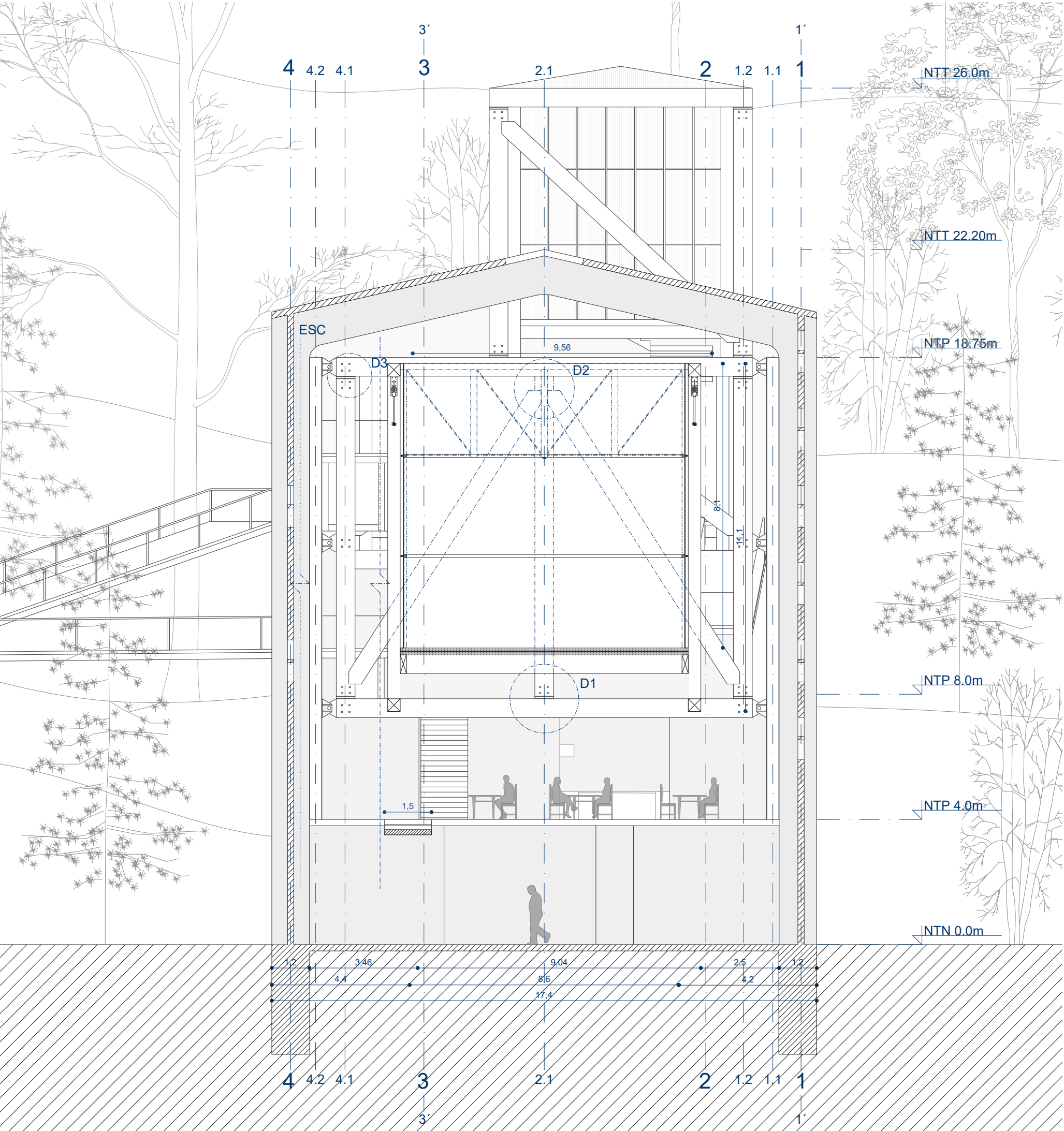
ESC. 1:125 CORTE A-A"
