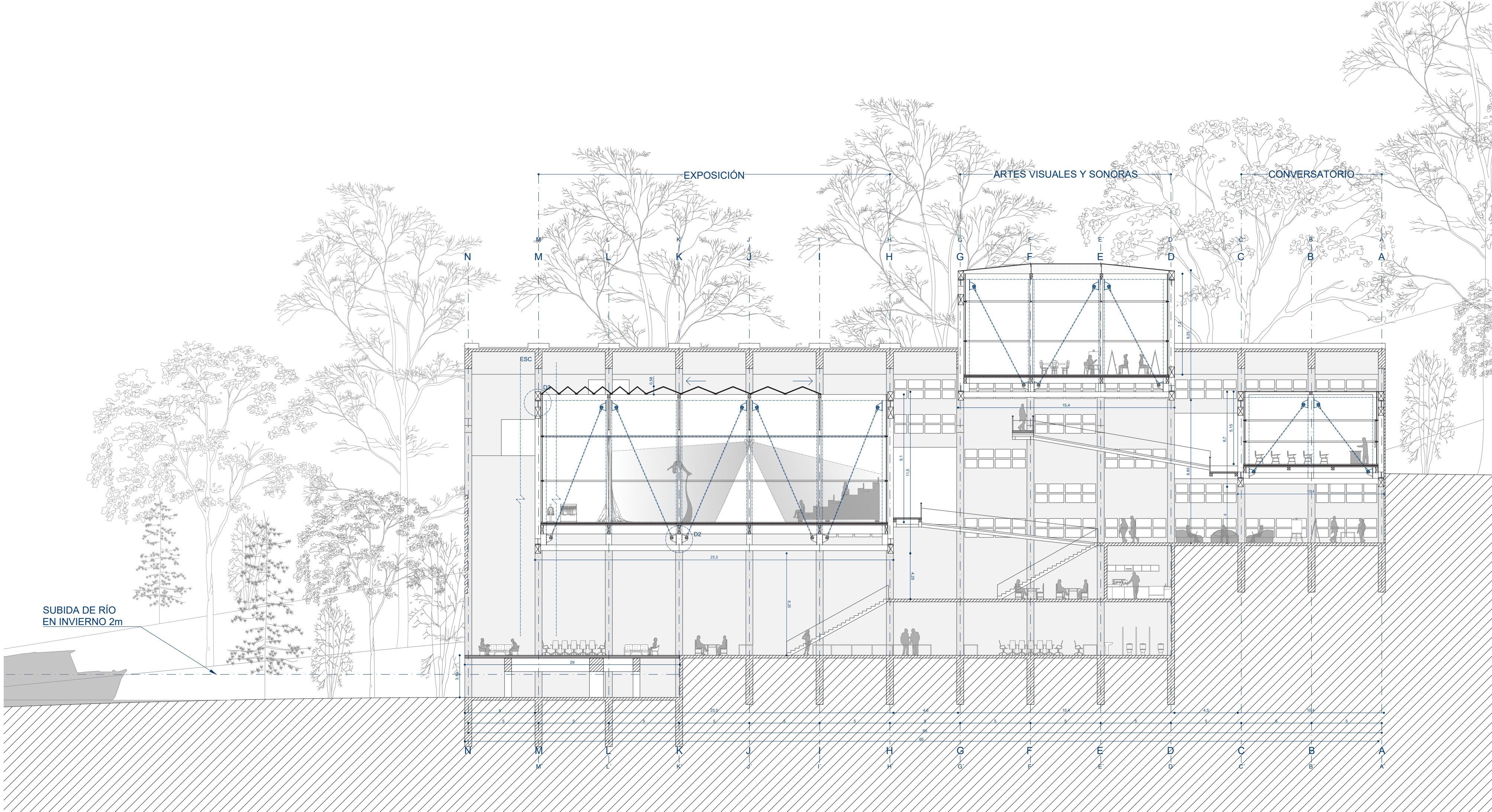
ESC. 1:200 CORTE B-B"
