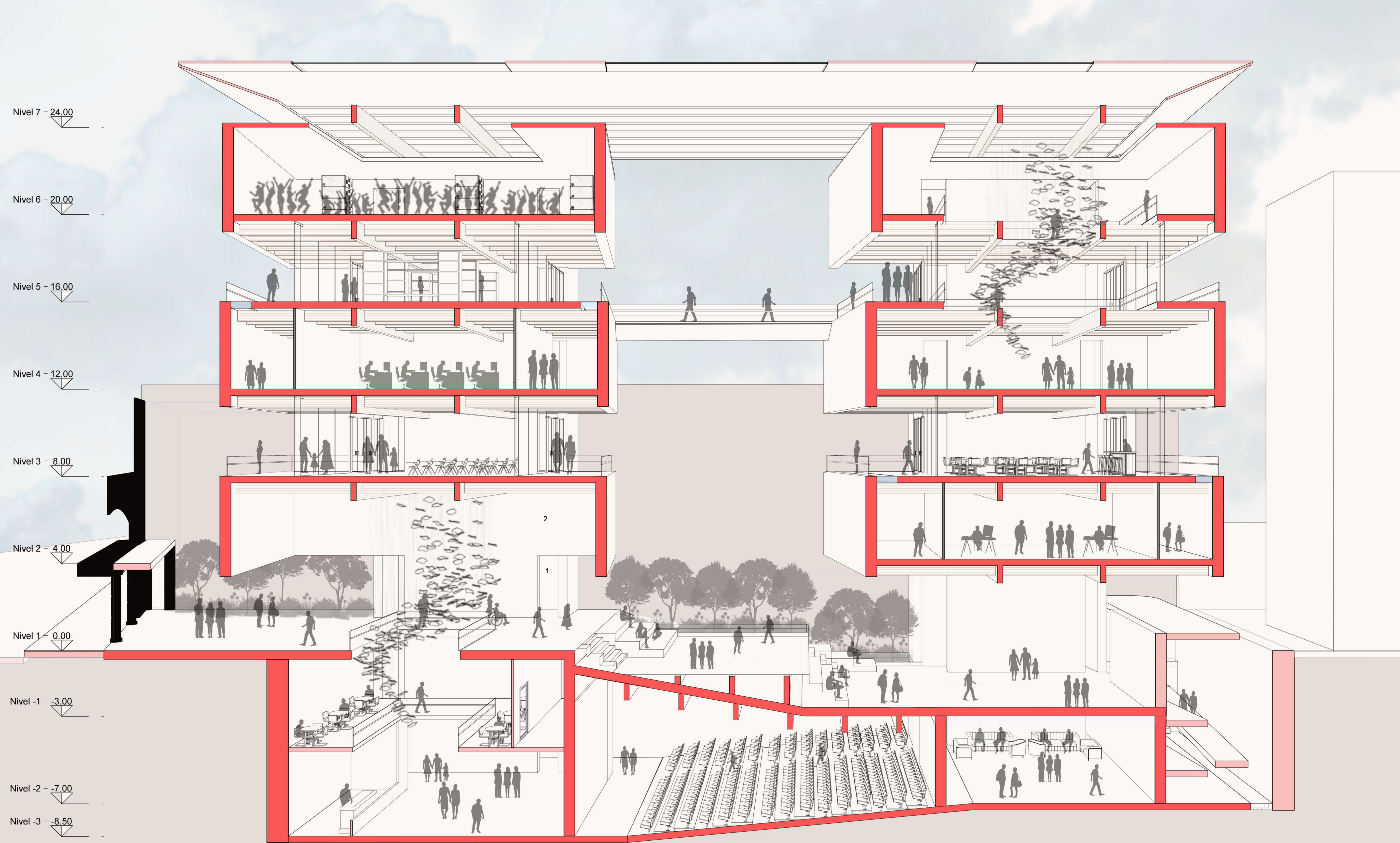
CORTE FUGADO A - A' ESC. 1:100
