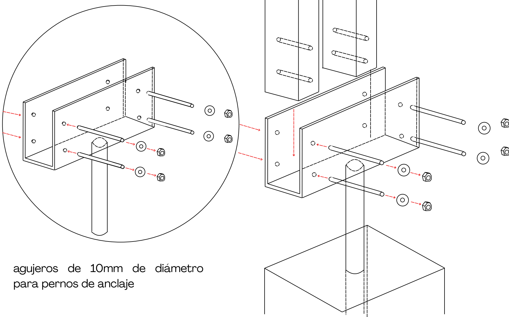
soporte galvanizado para postes 4" x 4"
